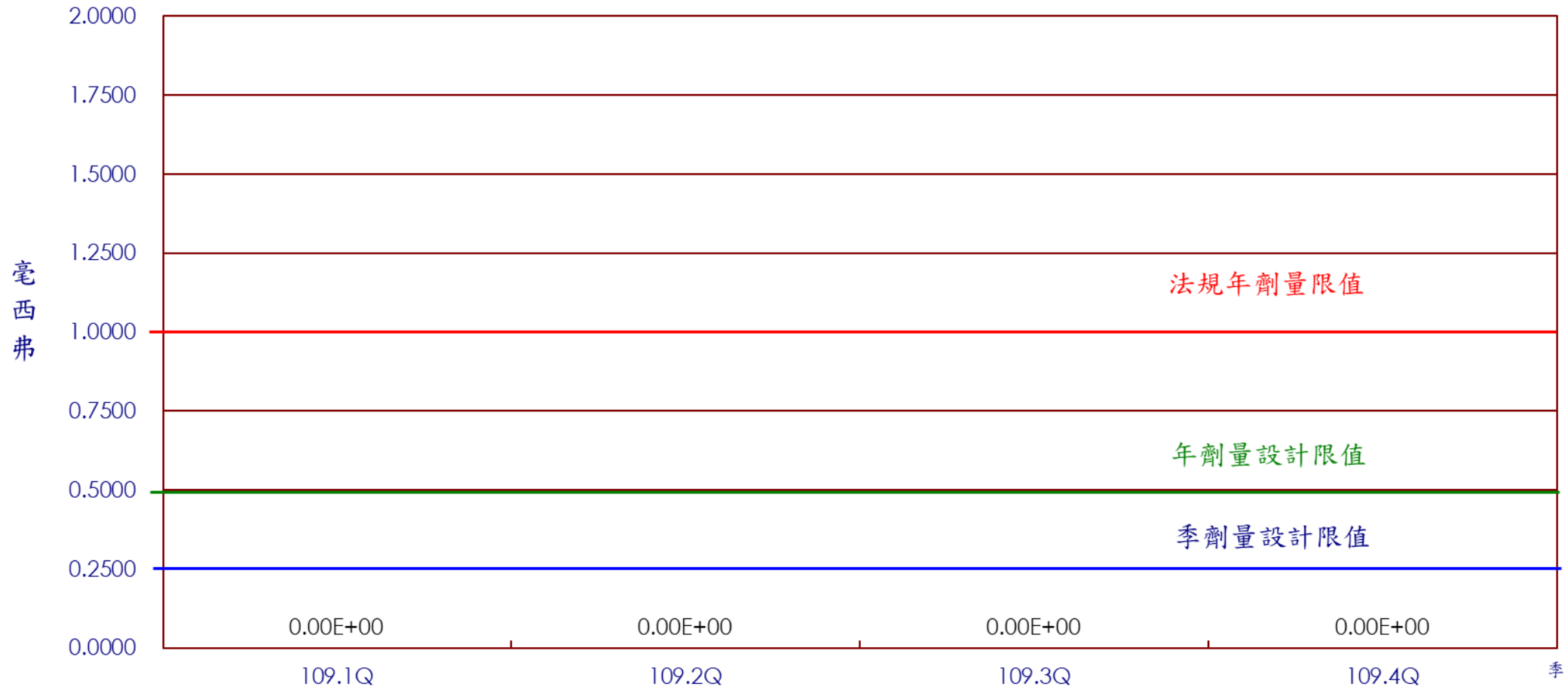
圖17 核能三廠109年第4季民眾最大個人全身劑量
