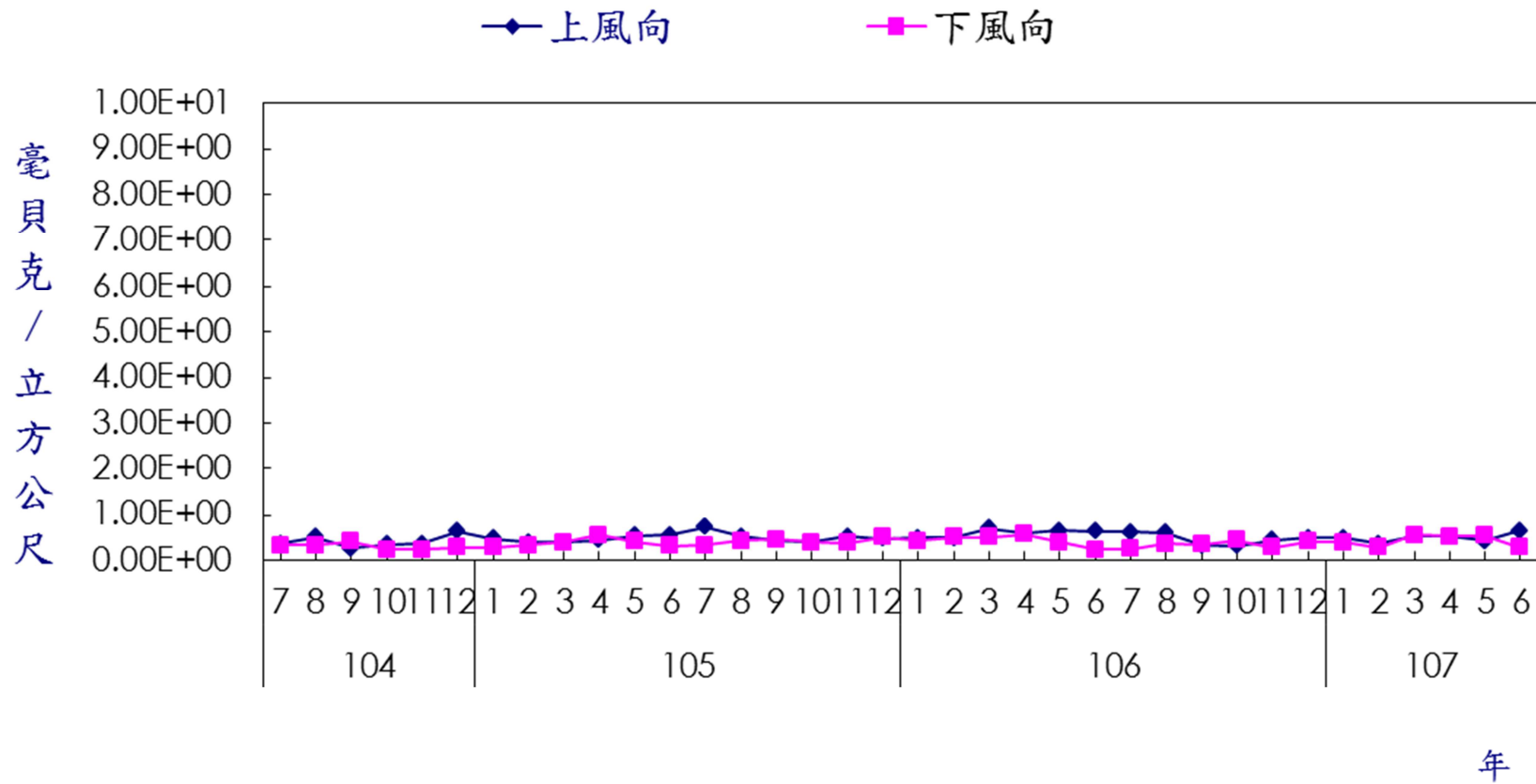
圖 15 核能三廠上下風向空氣微粒總貝他活度監測結果
