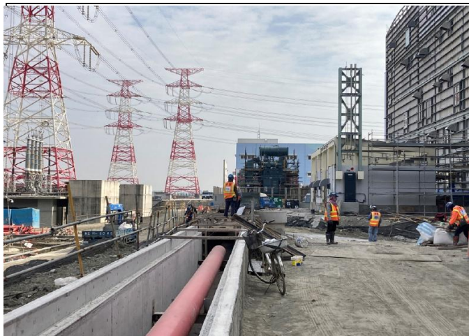
主發電設備工程 消防管溝施作
