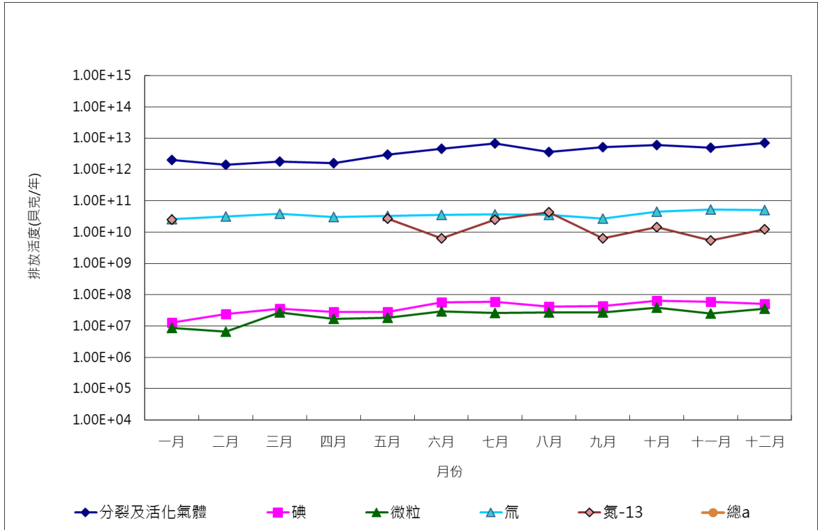
圖 8 108 年 1 號機放射性廢氣排放活度統計圖
