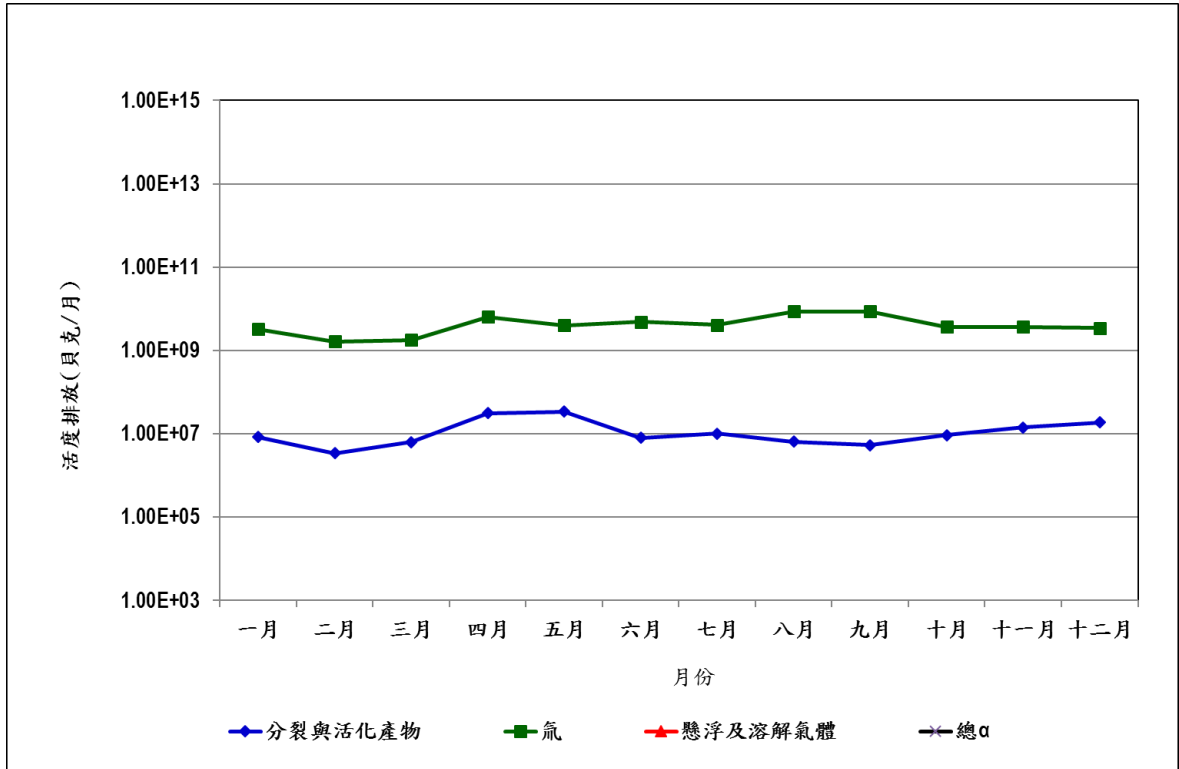
圖 10 108 年放射性廢水排放活度統計圖
