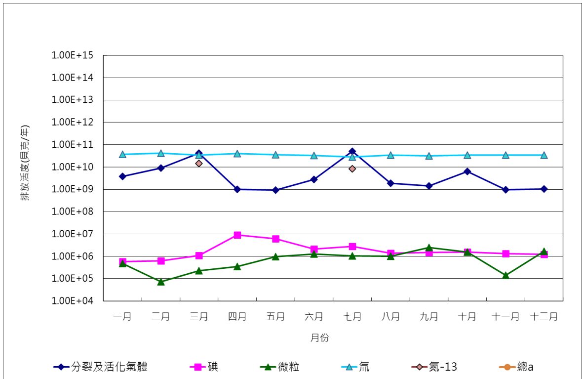
圖 9 108 年 2 號機放射性廢氣排放活度統計圖
