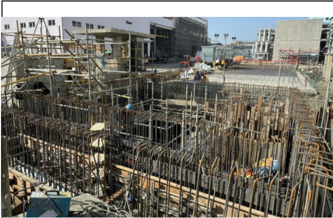
主發電設備工程 Unit 2 GT 廠房 結構體
