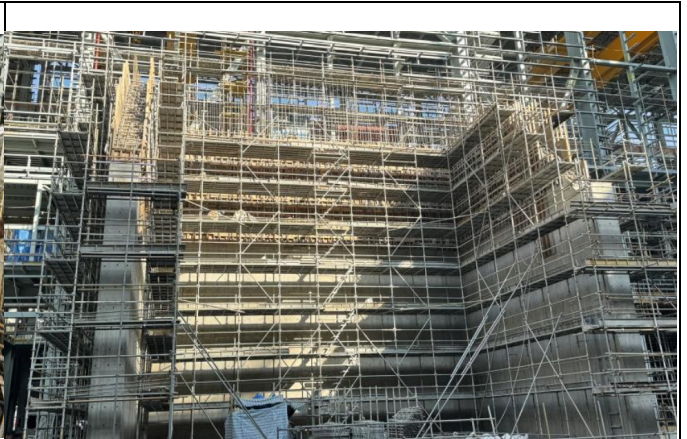
主發電設備工程 Unit 2 ST 變壓器 結構體
