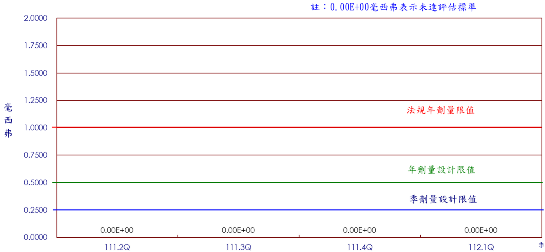
圖17 核能三廠112年第1季民眾最大個人全身劑量
