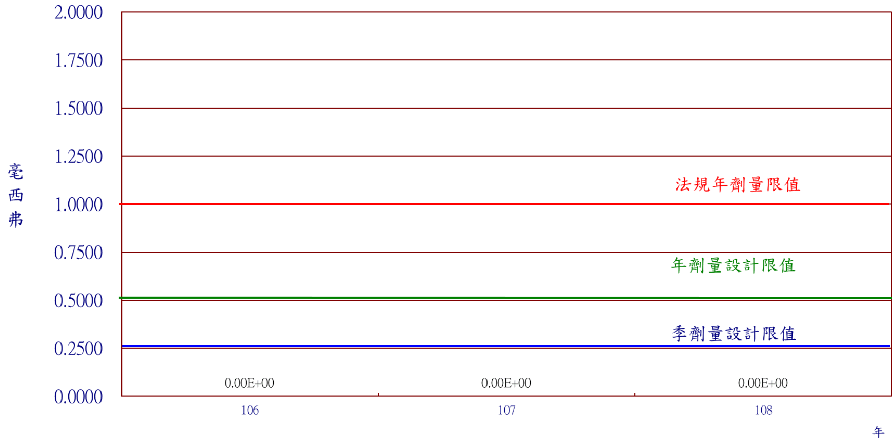
圖18 核能一廠108年民眾最大個人全身劑量
