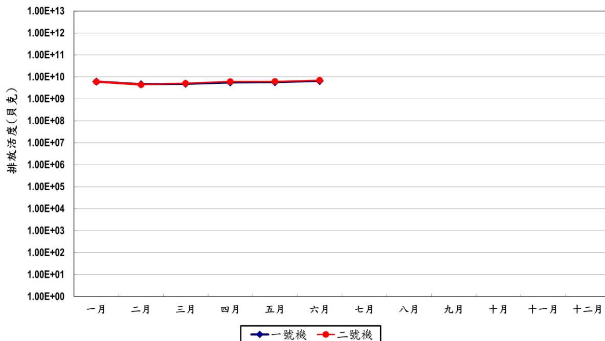
圖六 核二廠廢氣排放源-總排放活度統計圖
