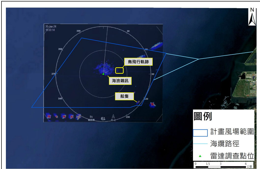
113 年 1 月 30 日 鳥類雷達調查回波圖
