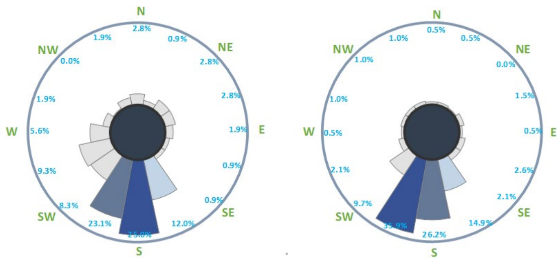
圖 2.2.3-3 112 年冬季水平雷達日間（左）及夜間（右）調查鳥類飛行方向
