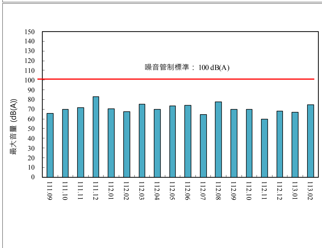
圖 3.1.1-1 歷次營建噪音均能音量值及最大音量值變化圖
