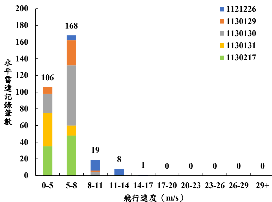
圖 2.2.4-1 112 年冬季水平雷達調查追蹤距離超過 1 公里軌跡之飛行速度
