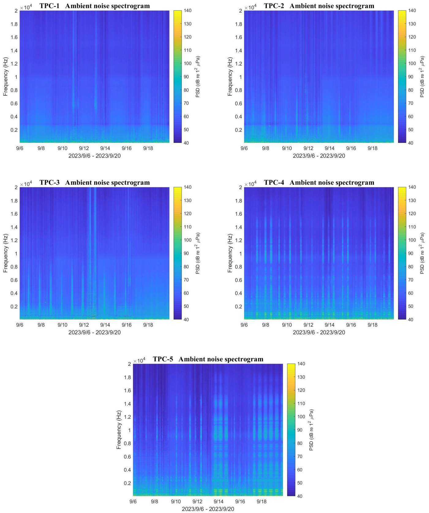
圖 2.8-2 本計畫風場 TPC-1~TPC-5 環境噪音時頻譜圖
