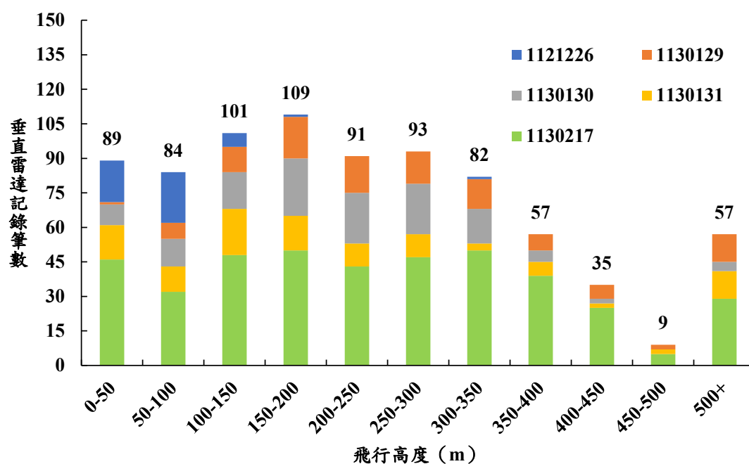
圖 2.2.2-1 112 年冬季垂直雷達調查高度分佈
