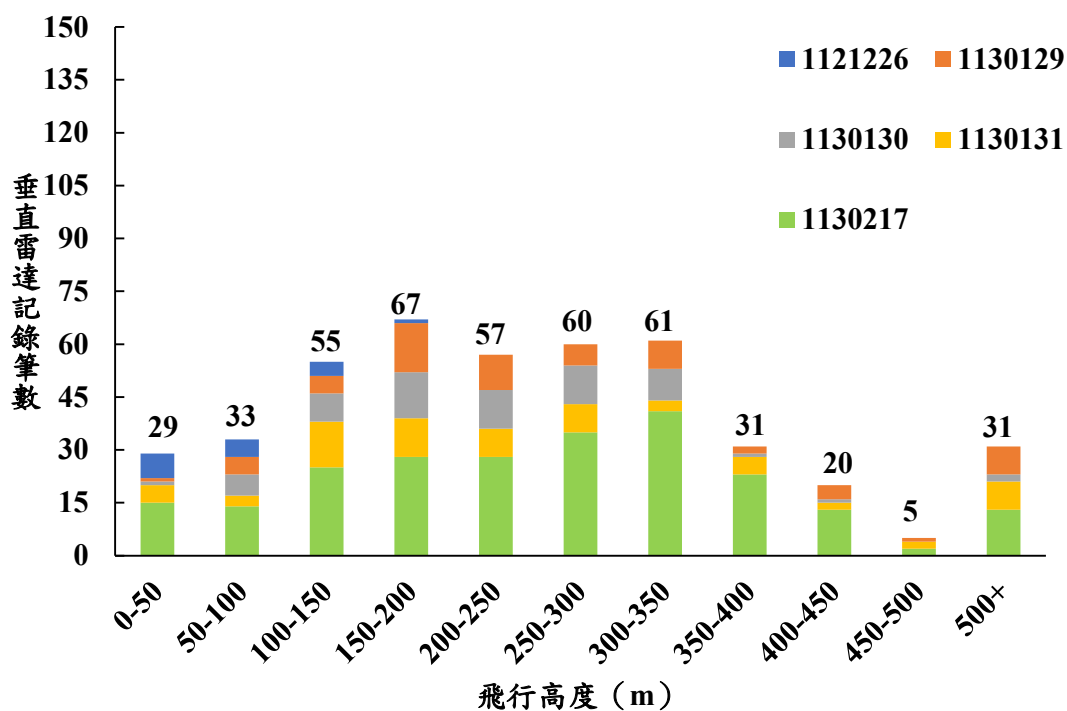
圖 2.2.2-3 112 年冬季垂直雷達夜間調查高度分佈
