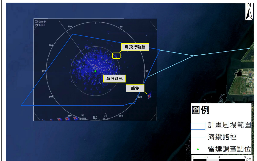
113 年 1 月 29 日鳥類雷達調查回波圖
