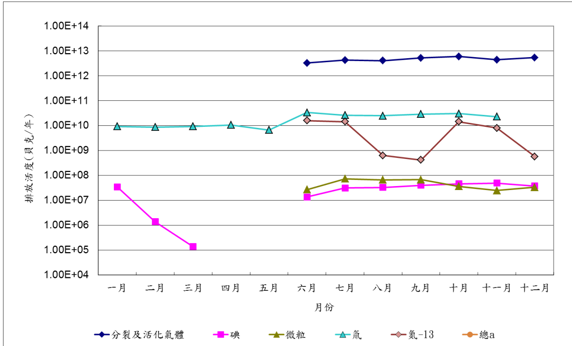
圖 8 106 年一號機放射性廢氣排放活度統計圖
