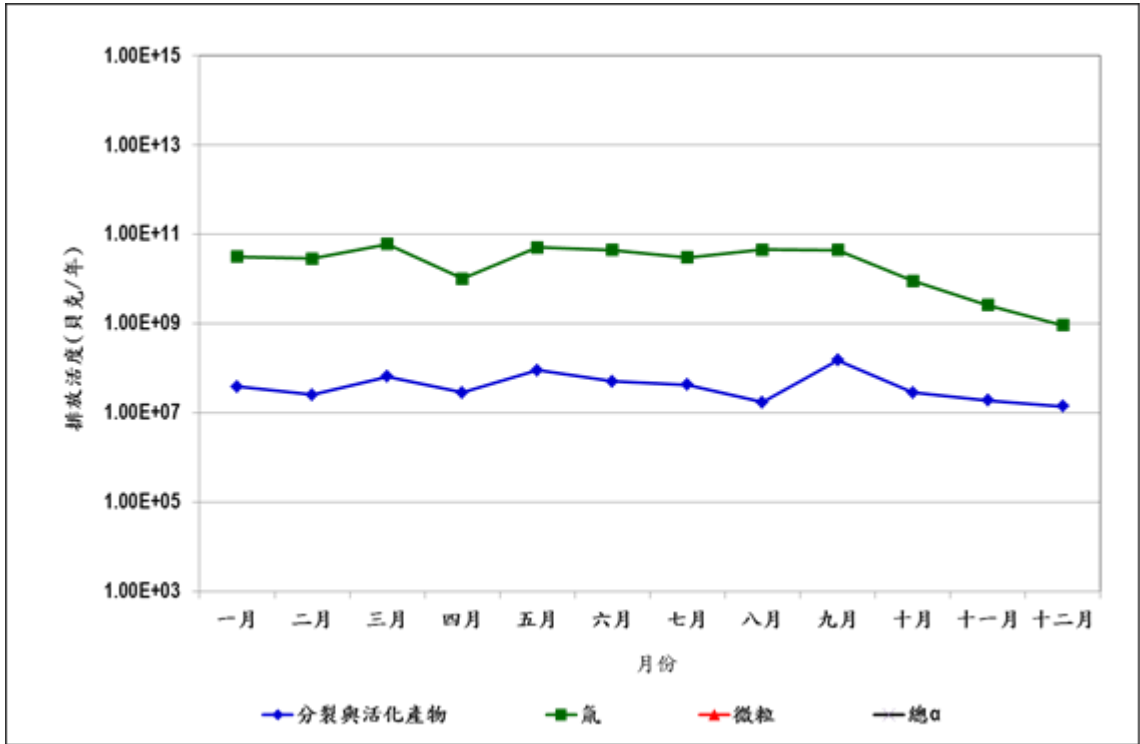
圖 10 106 年放射性廢水排放活度統計圖
