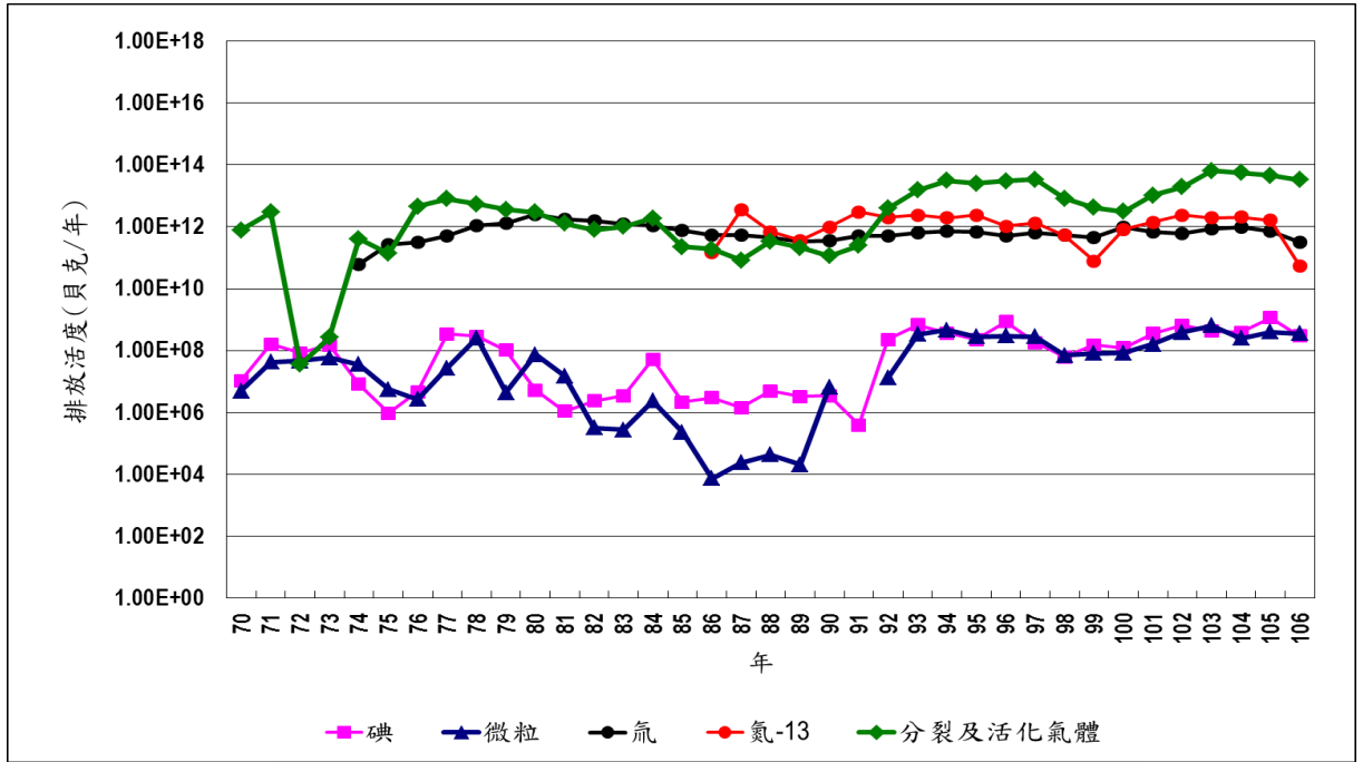
圖 6 歷年放射性廢氣排放活度趨勢圖
