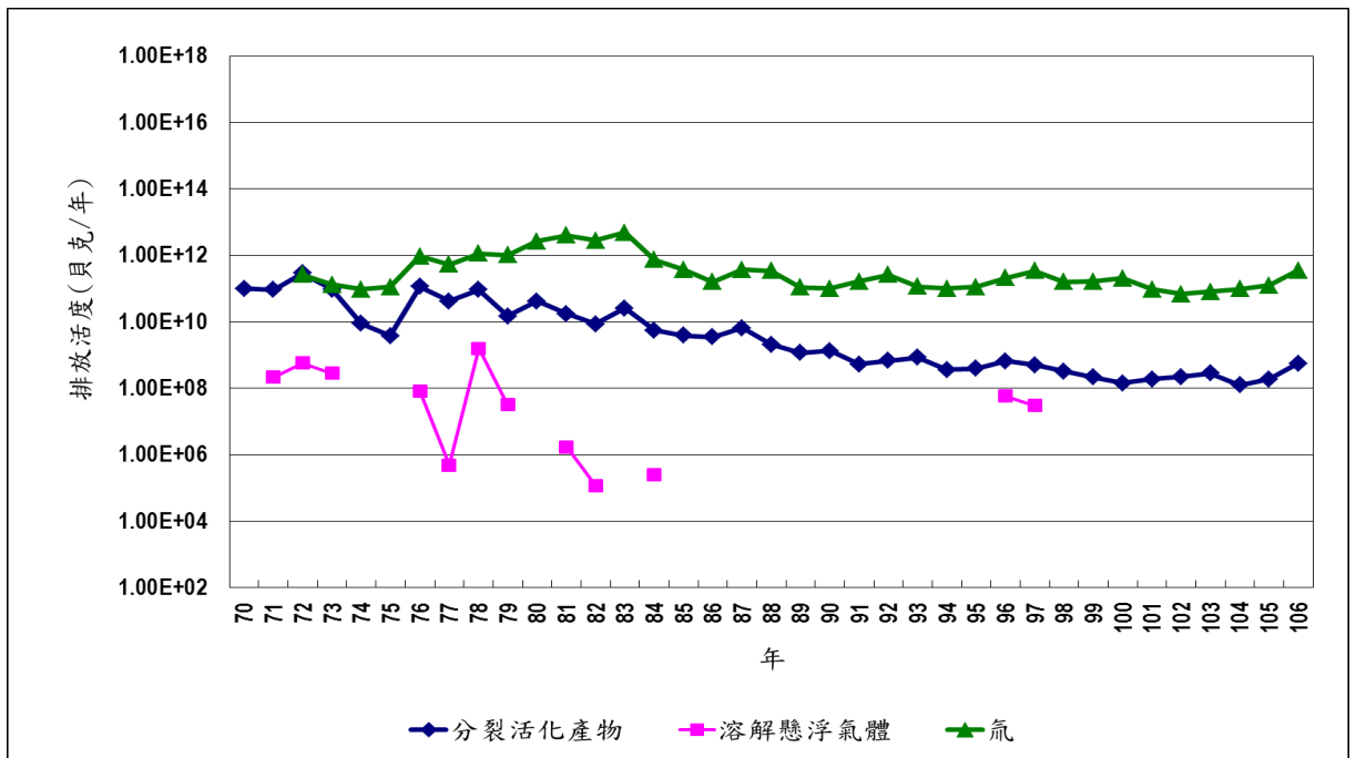
圖 7 歷年放射性廢水排放活度趨勢圖
