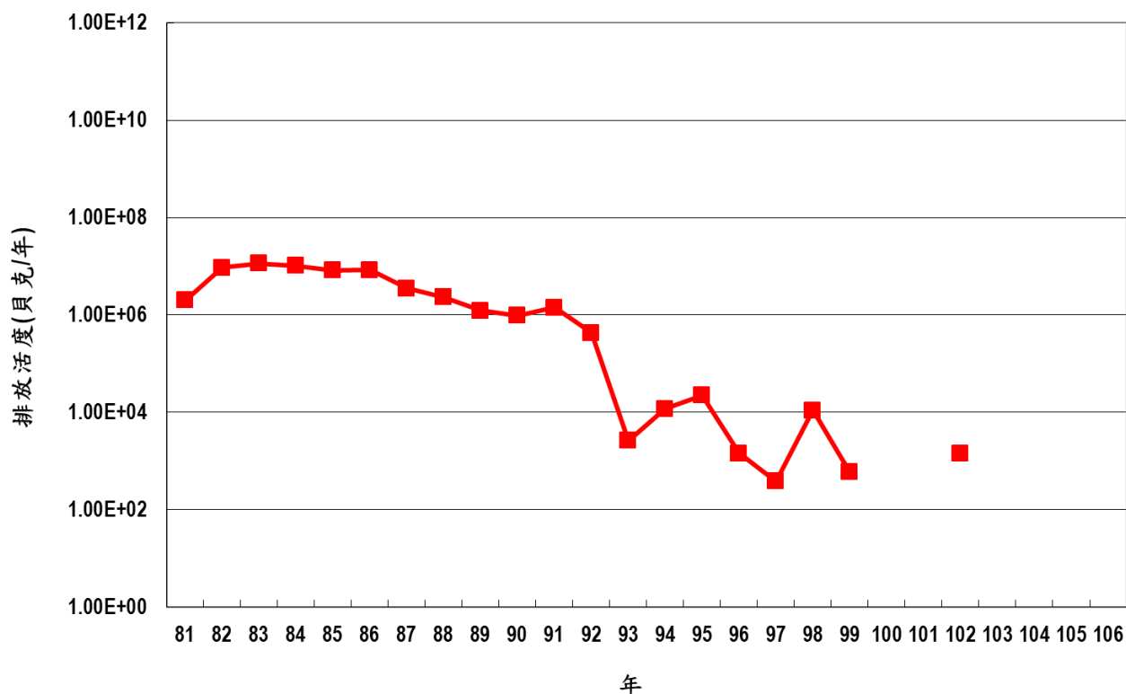
圖 3 歷年放射性廢氣排放活度統計圖
