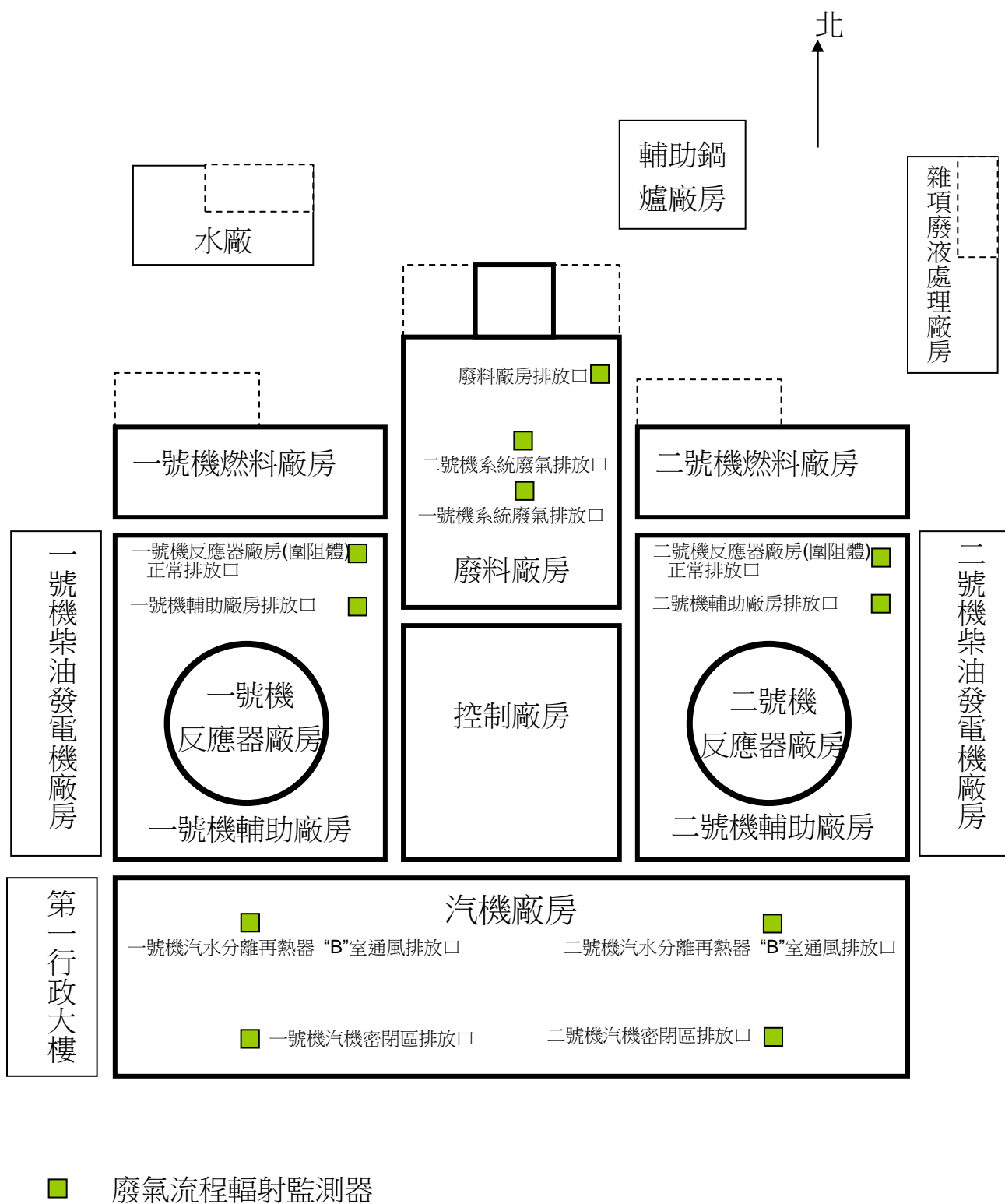
圖 4 放射性廢氣排放口監測位置圖
