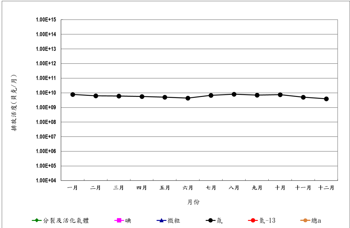
圖 8 112 年 1 號機放射性廢氣排放活度統計圖
