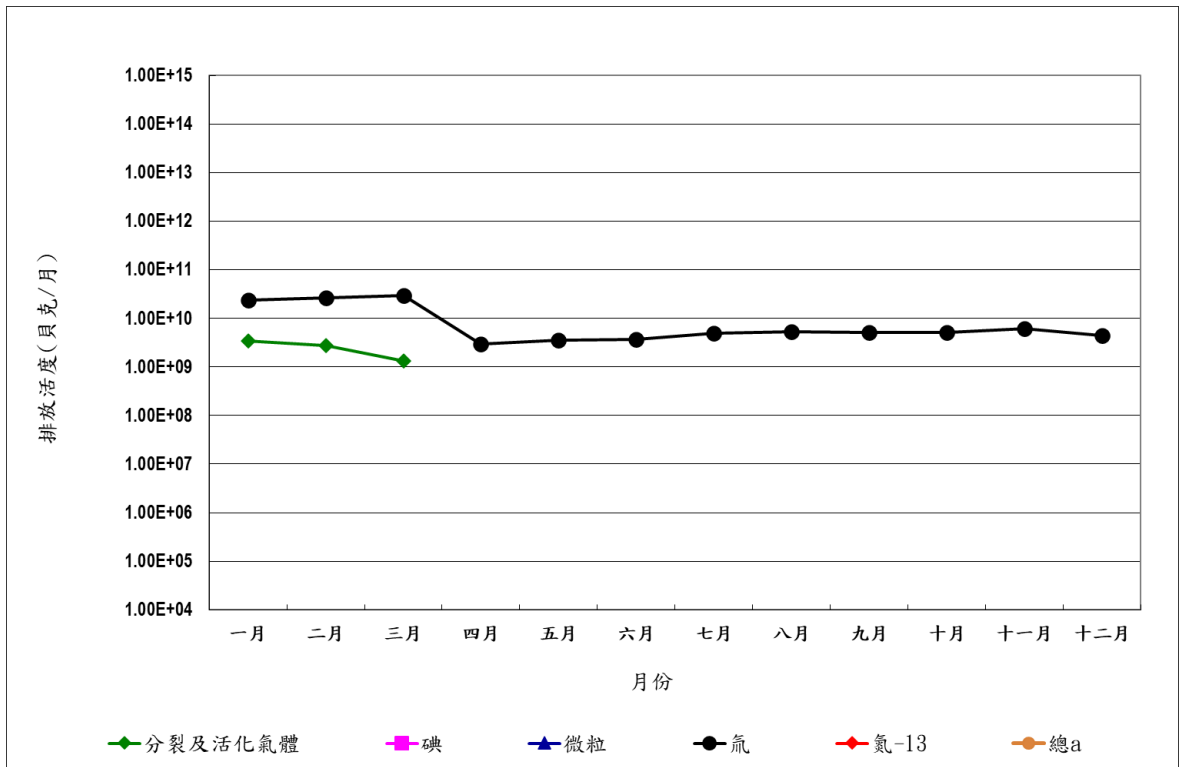
圖 9 112 年 2 號機放射性廢氣排放活度統計圖
