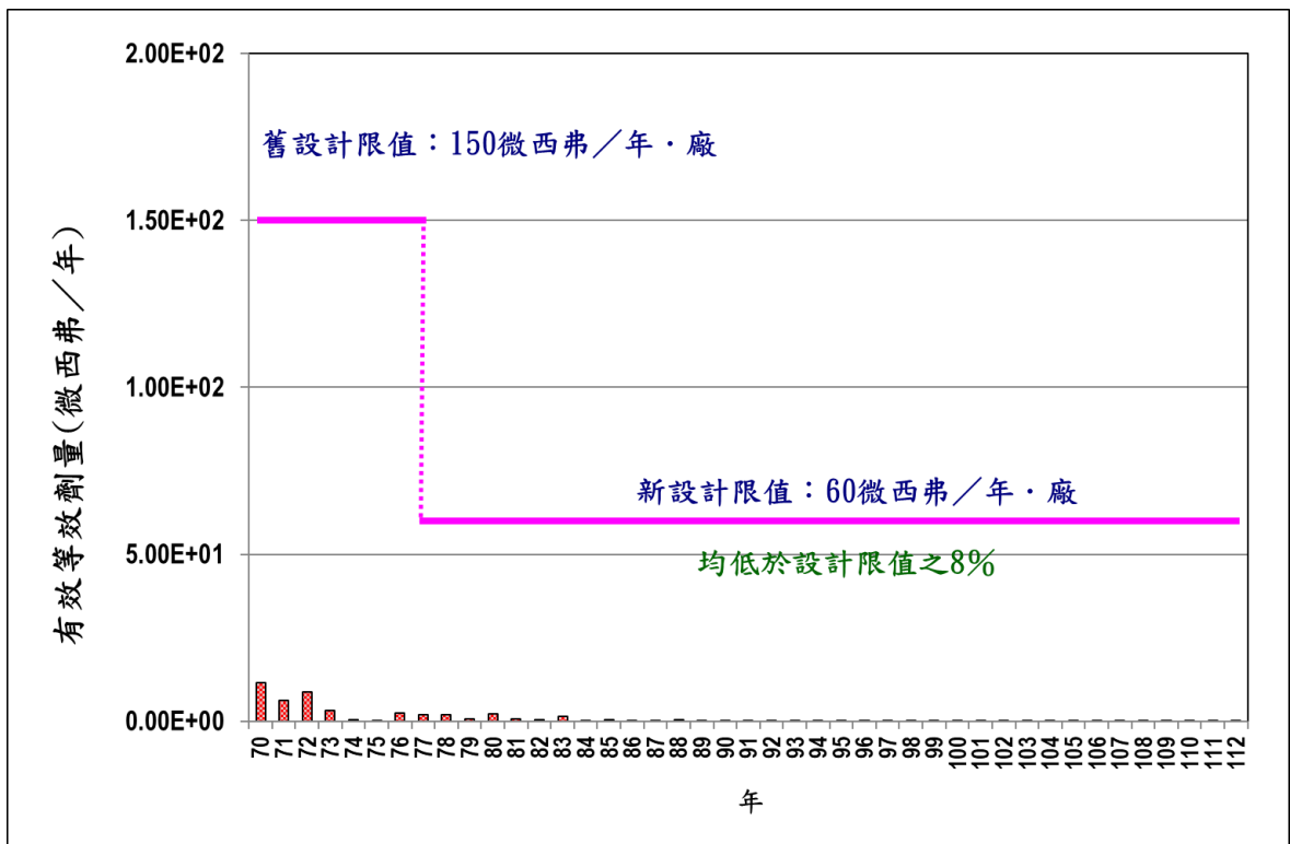
圖 16 歷年放射性廢水排放造成關鍵群體有效劑量趨勢圖
