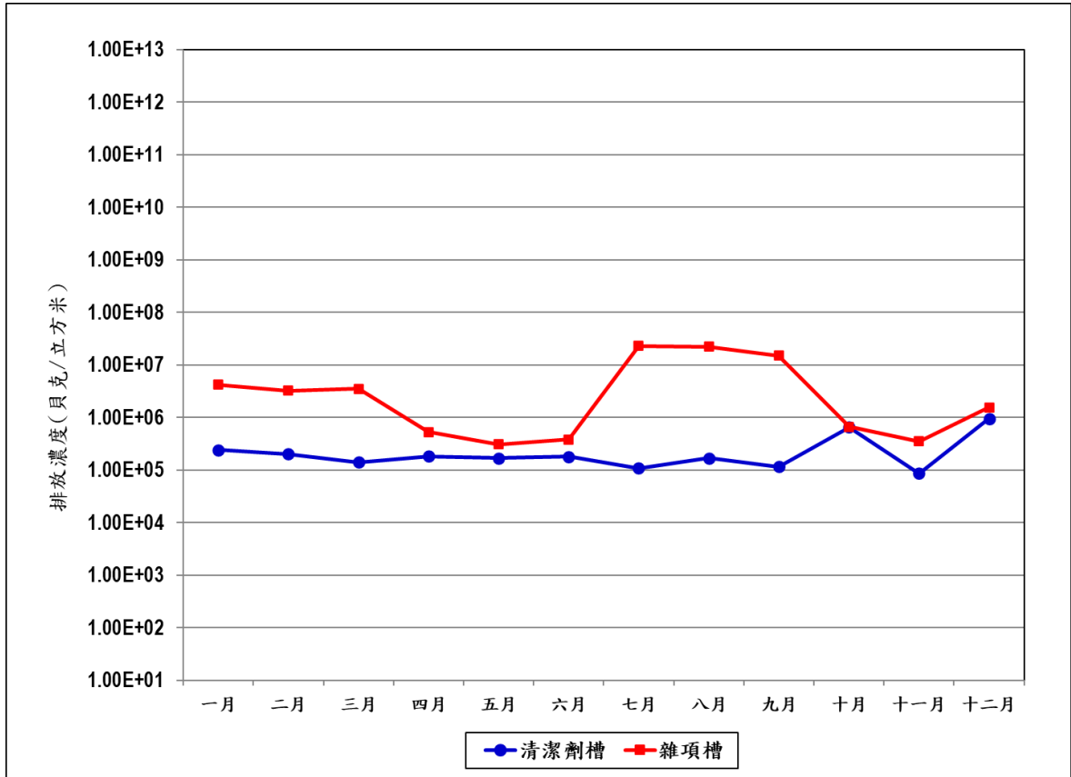
圖 14 112 年各廢水排放源總排放濃度統計圖
