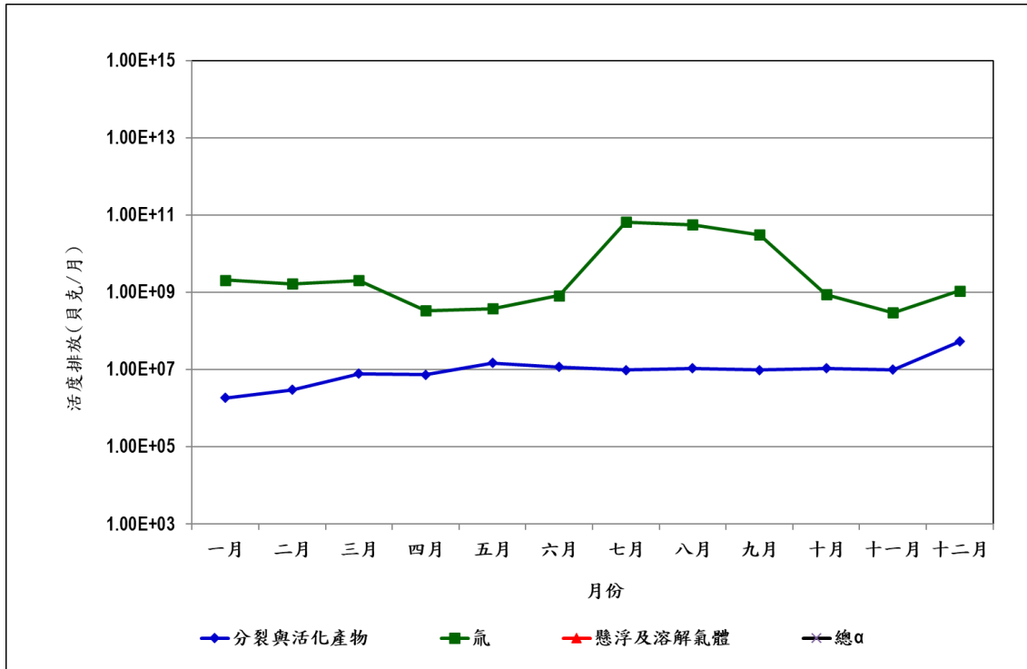
圖 12 112 年放射性廢水排放活度統計圖
