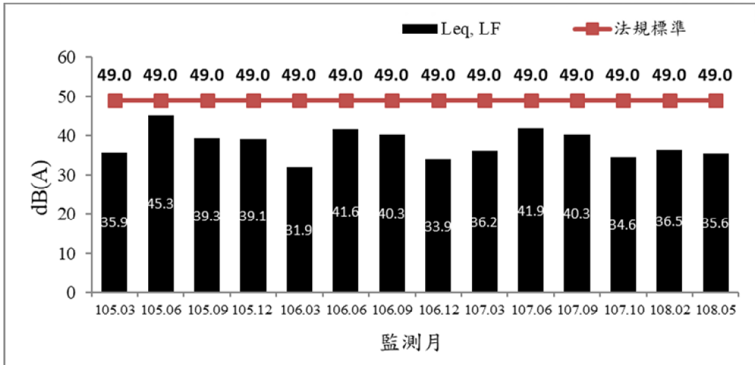
圖 2.4-1 低頻噪音監測結果圖
