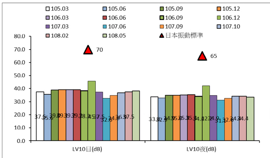
圖 2.2-2 計畫基地振動監測結果圖
