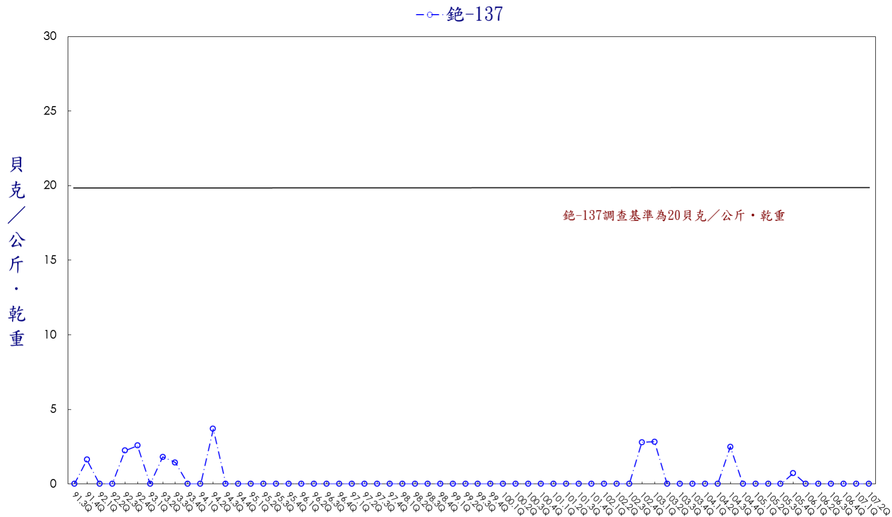
圖4 低放貯存場排水口岸砂(SS502)加馬能譜分析結果
