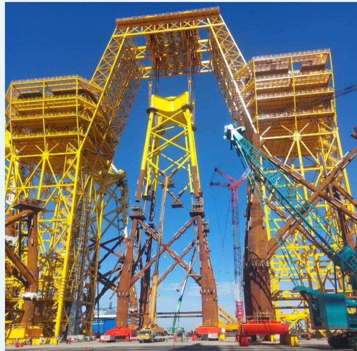
風力發電機水下基礎套筒桁架
