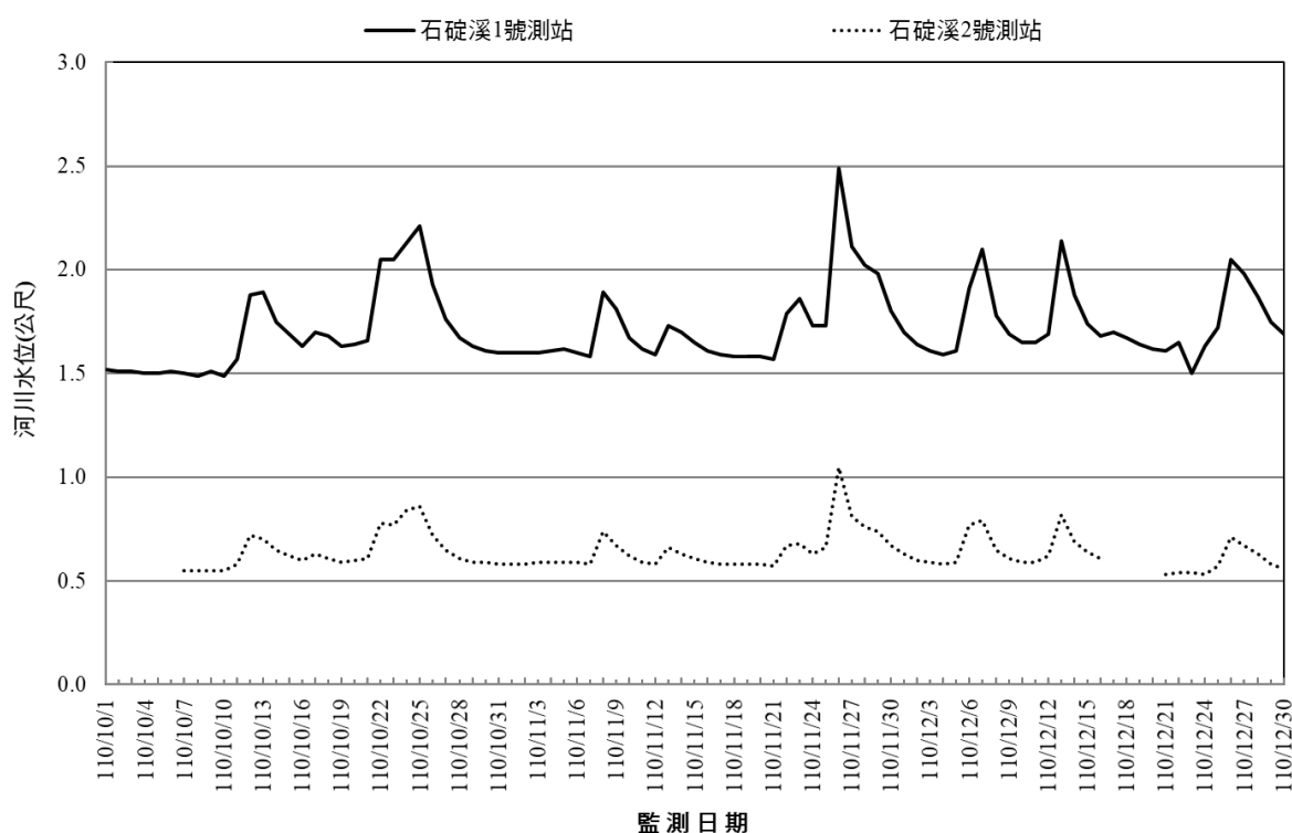
圖 2.2-1 核四封存期間河川水文 110 年 10~12 月水位變化圖
