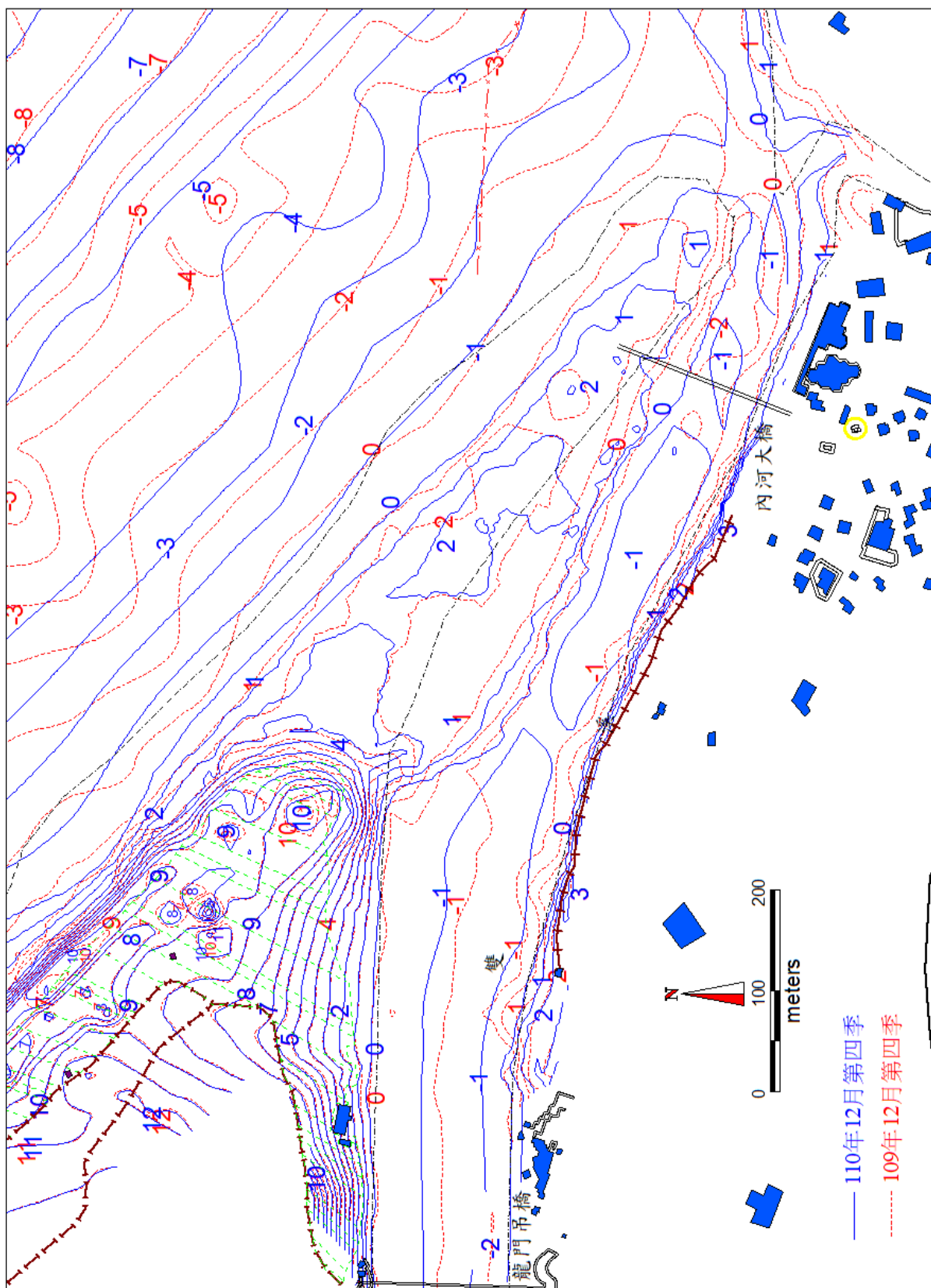
圖 3.1-12 核四環境監測海岸地形福隆附近 110 年 12 月與 109 年 12 月監測結果比較
