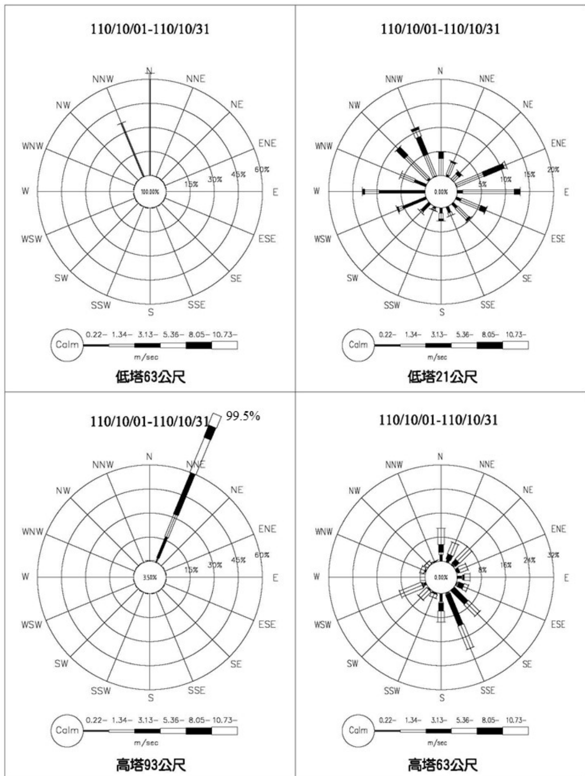
圖 2.1-1 核四封存期間環境監測氣象塔 110 年 10 月風花圖
