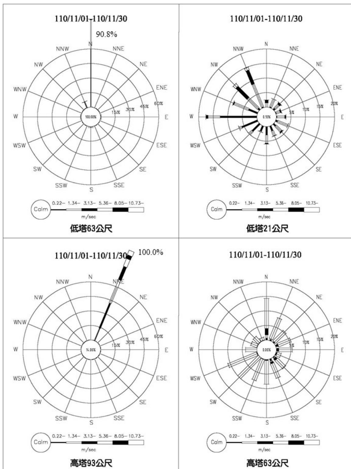
圖 2.1-2 核四封存期間環境監測氣象塔 110 年 11 月風花圖
