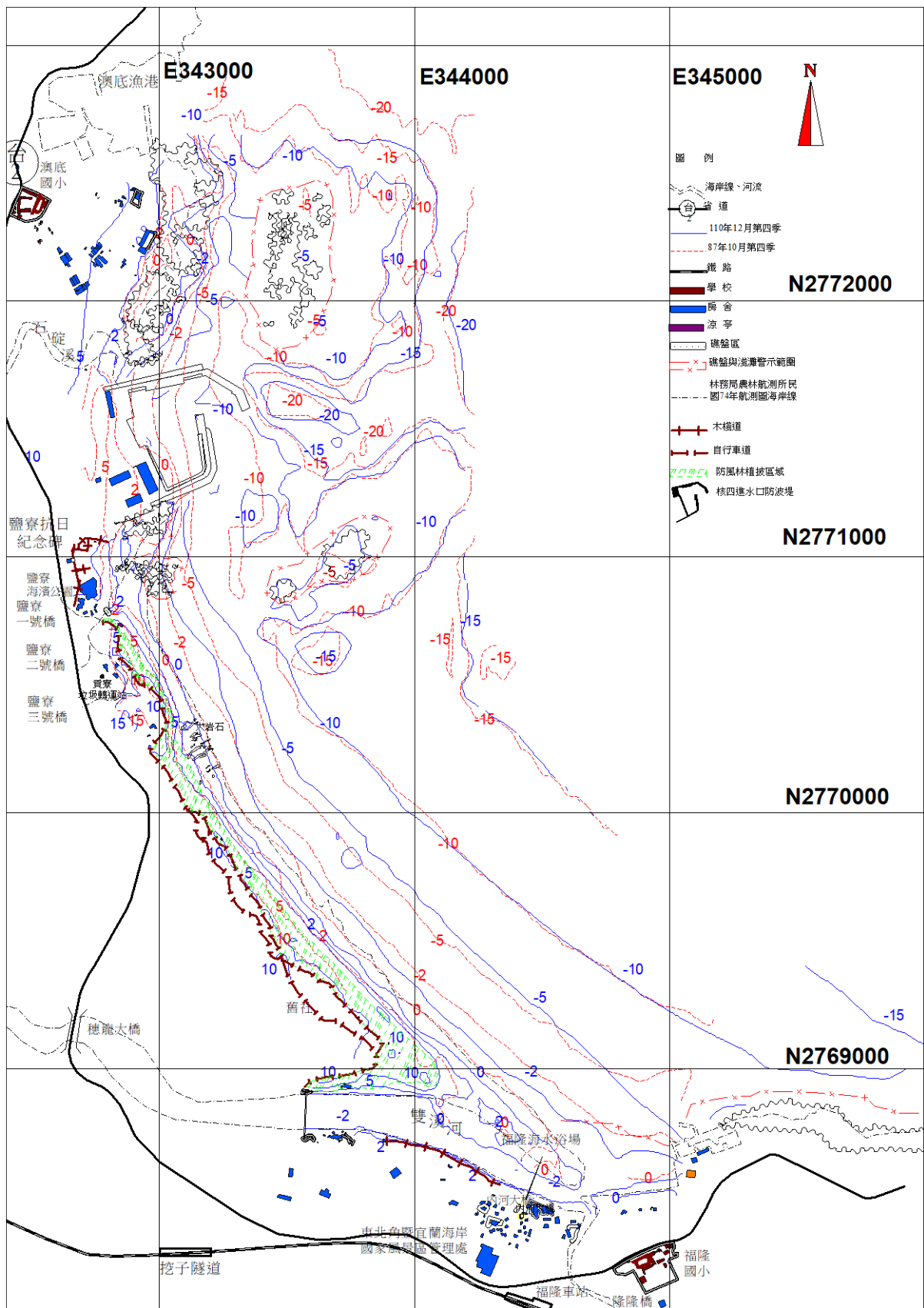
圖 3.1-13 核四環境監測海岸地形 110 年 12 月與 87 年 10 月（海事工程施工前）監測結果比較
