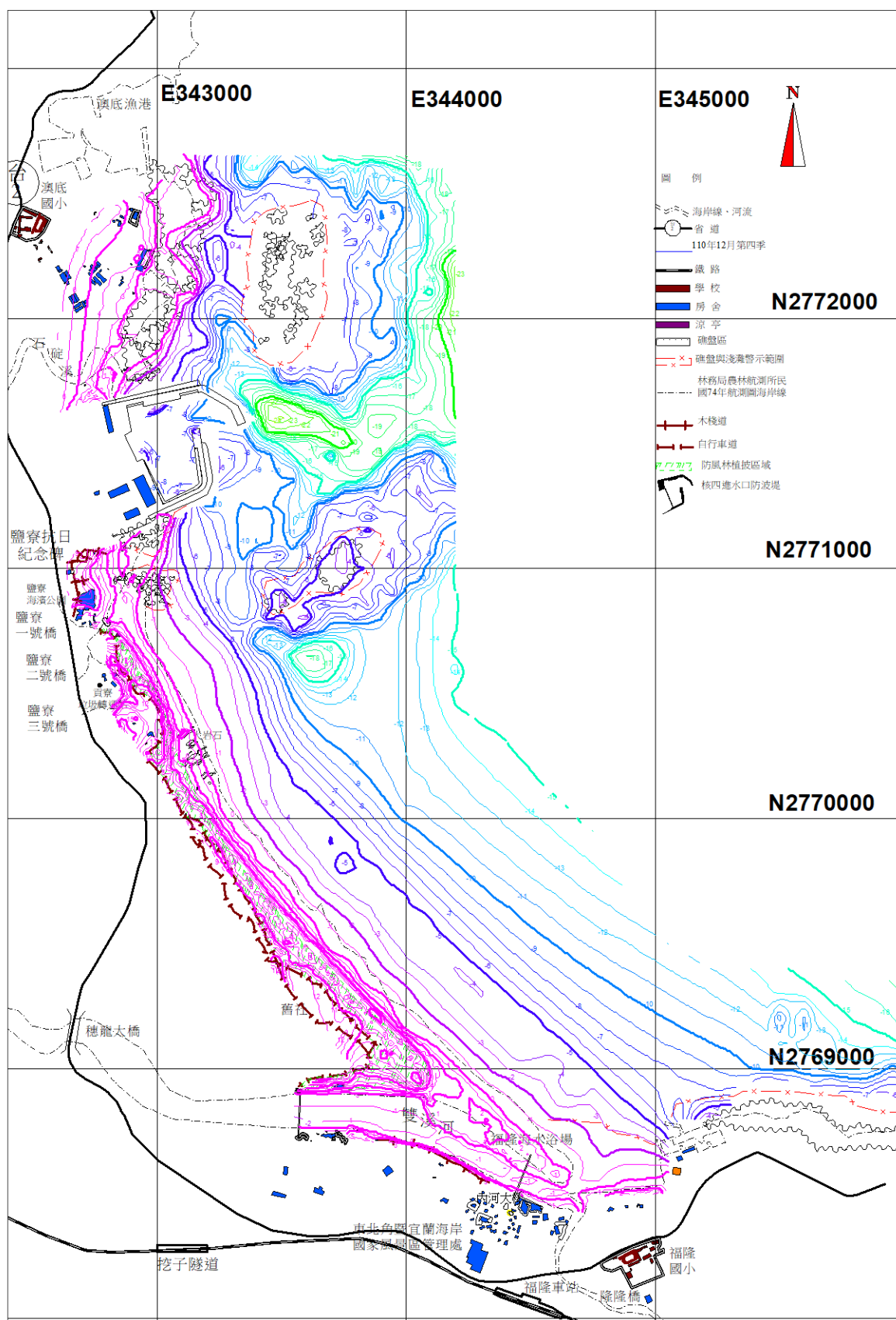
圖 2.5-2 核四封存期間環境監測海岸地形 110 年第 4 季 海岸地形監測結果
