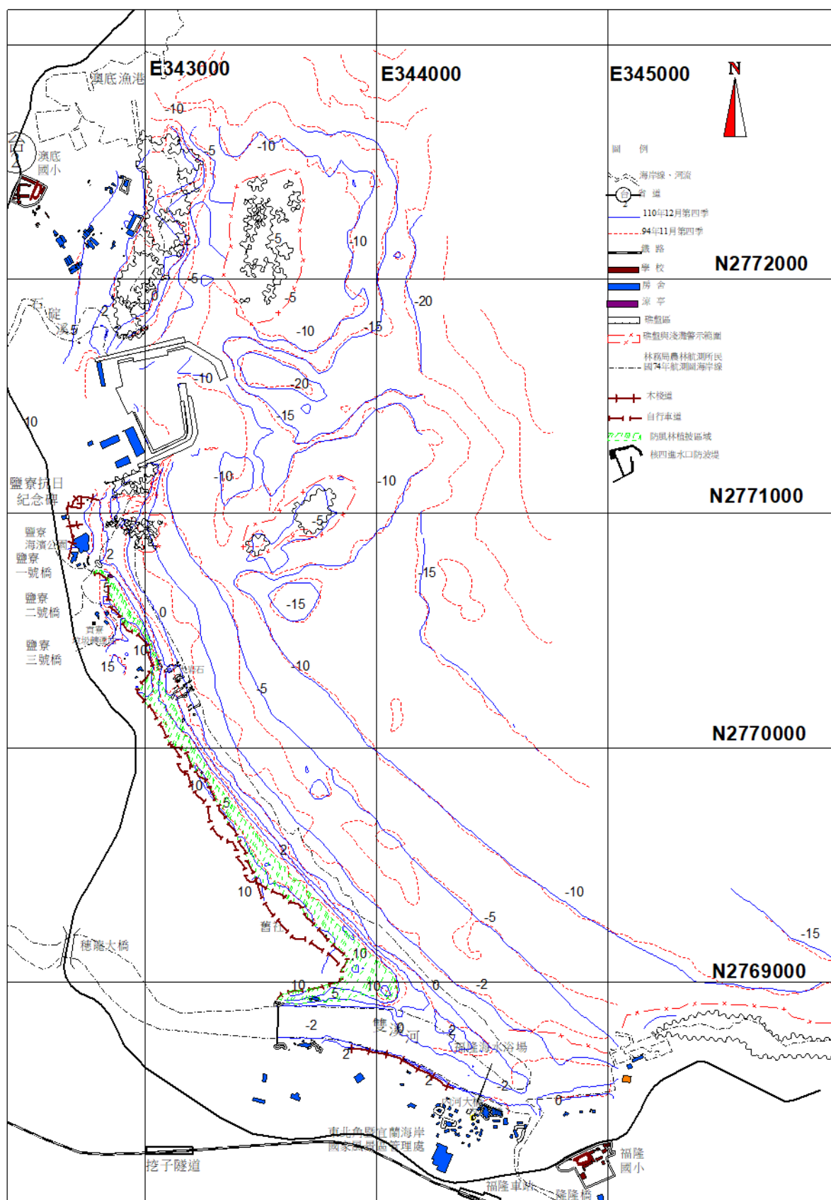
圖 3.1-14 核四環境監測海岸地形 110 年 12 月與 94 年 11 月（海事工程完工後）監測結果比較
