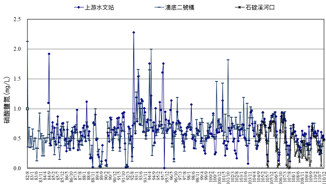
圖 3.1-7 核四環境監測河川水質歷年調查硝酸鹽氮濃度變化圖
