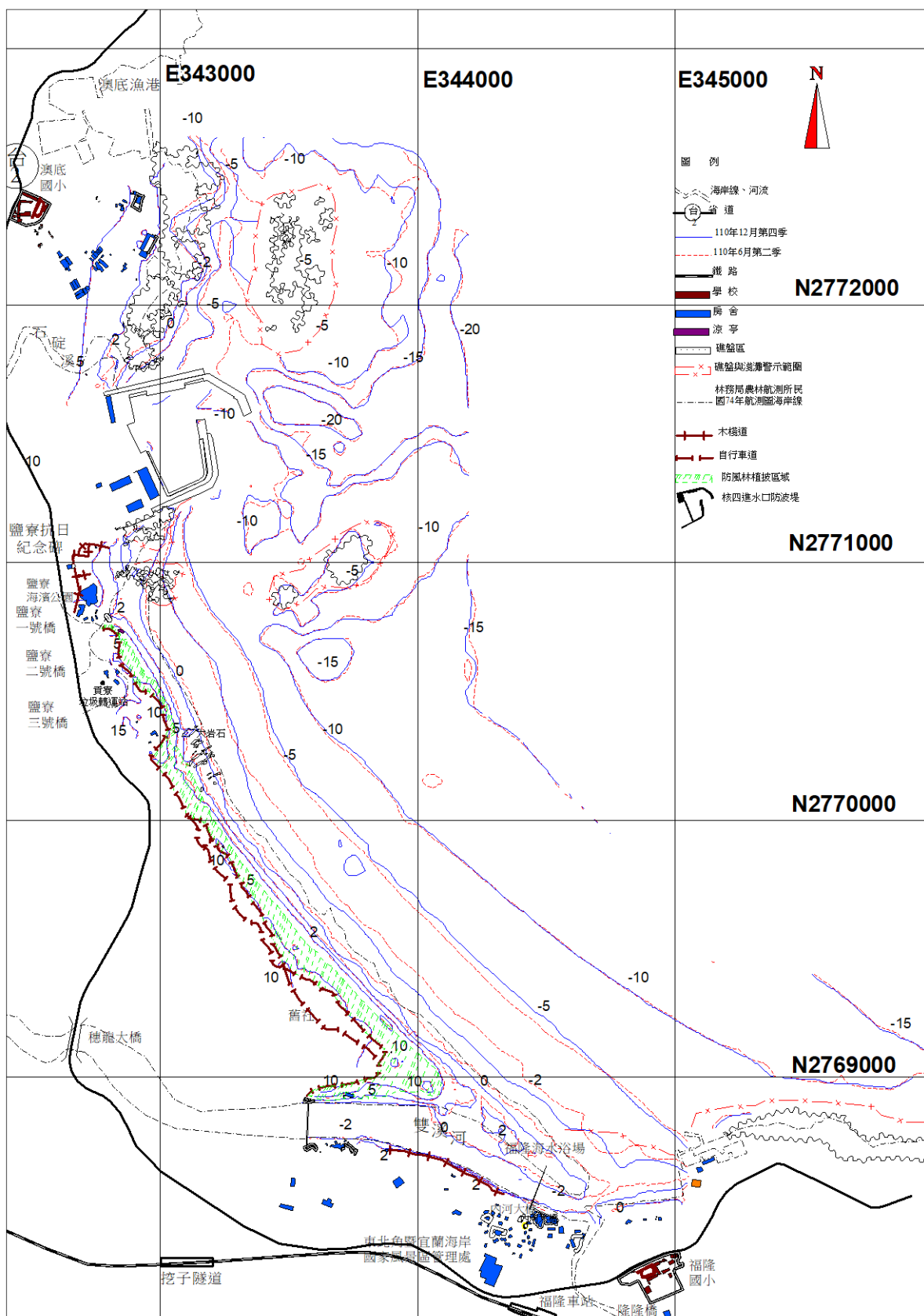
圖 2.5-5 核四封存期間海岸地形 110 年第 4 季與 110 年第 2 季監測結果比較
