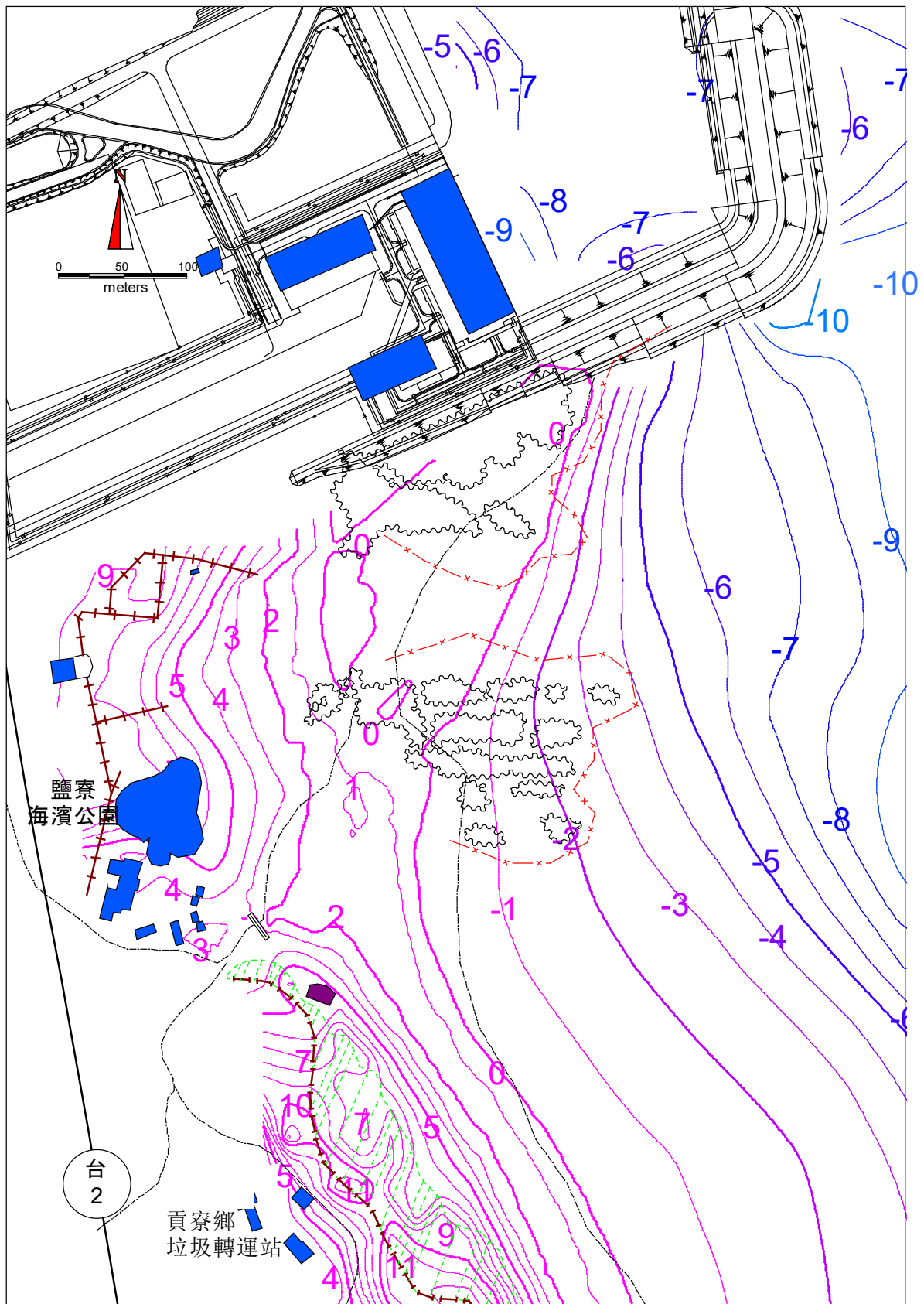
圖 2.5-3 核四封存期間鹽寮公園附近 110 年第 4 季 海岸地形監測結果
