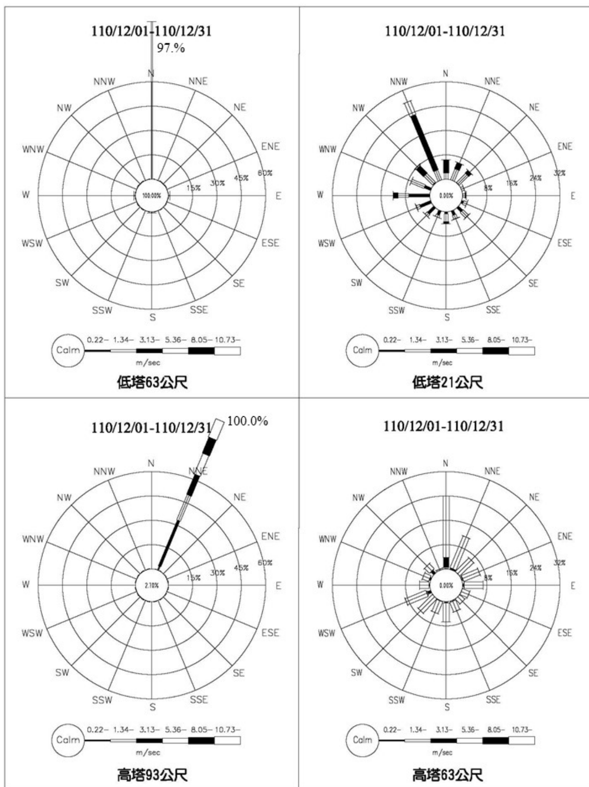
圖 2.1-3 核四封存期間環境監測氣象塔 110 年 12 月風花圖
