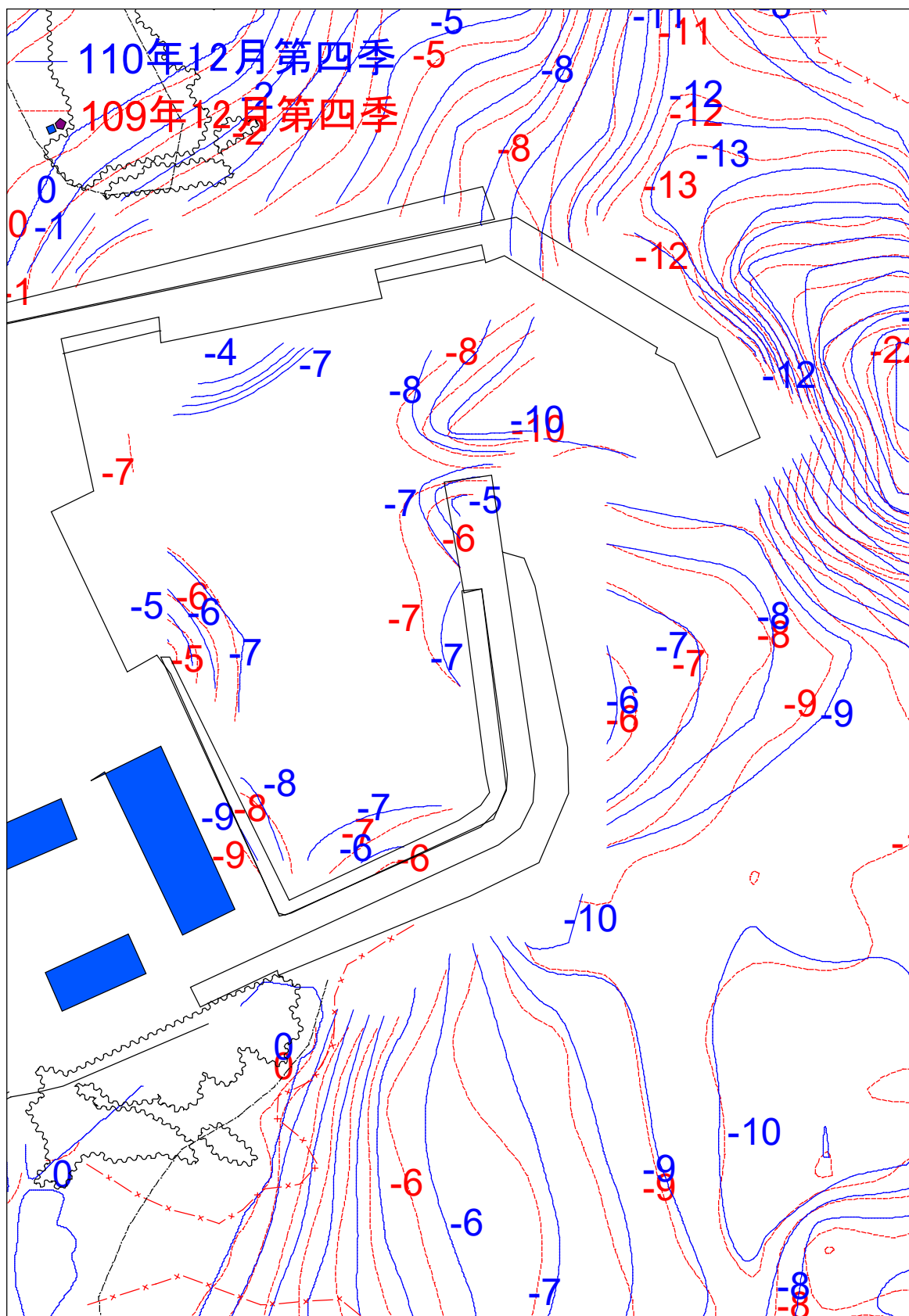
圖 3.1-11 核四環境監測海岸地形進水口防坡堤 110 年 12 月與 109 年 12 月監測結果比較
