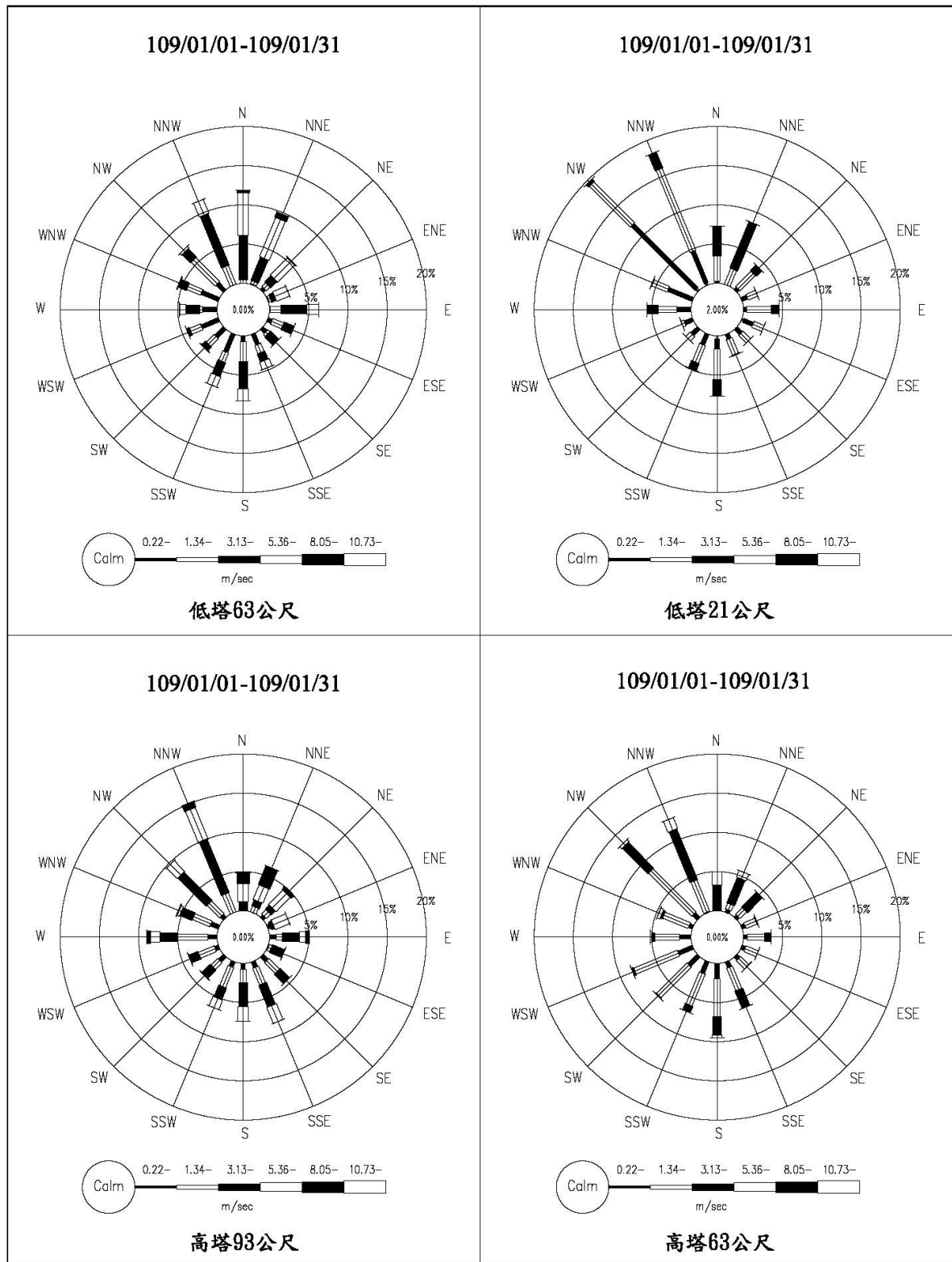
圖 2.1-1 核四封存期間環境監測氣象塔 109 年 1 月風花圖
