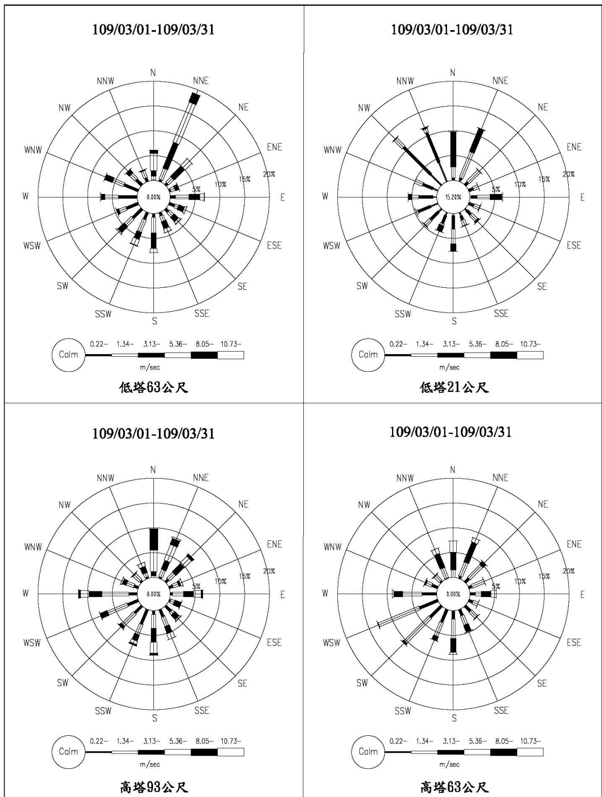
圖 2.1-2 核四封存期間環境監測氣象塔 109 年 3 月風花圖
