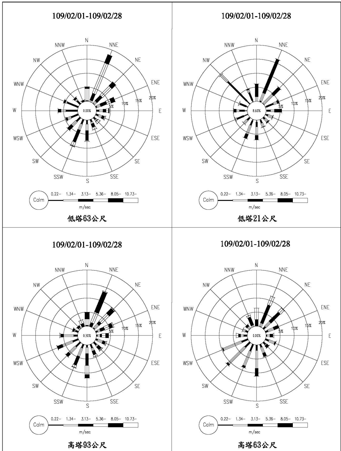
圖 2.1-2 核四封存期間環境監測氣象塔 109 年 2 月風花圖
