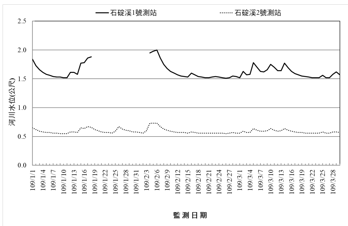
圖 2.2-1 核四封存期間河川水文 109 年 1~3 月水位變化圖
