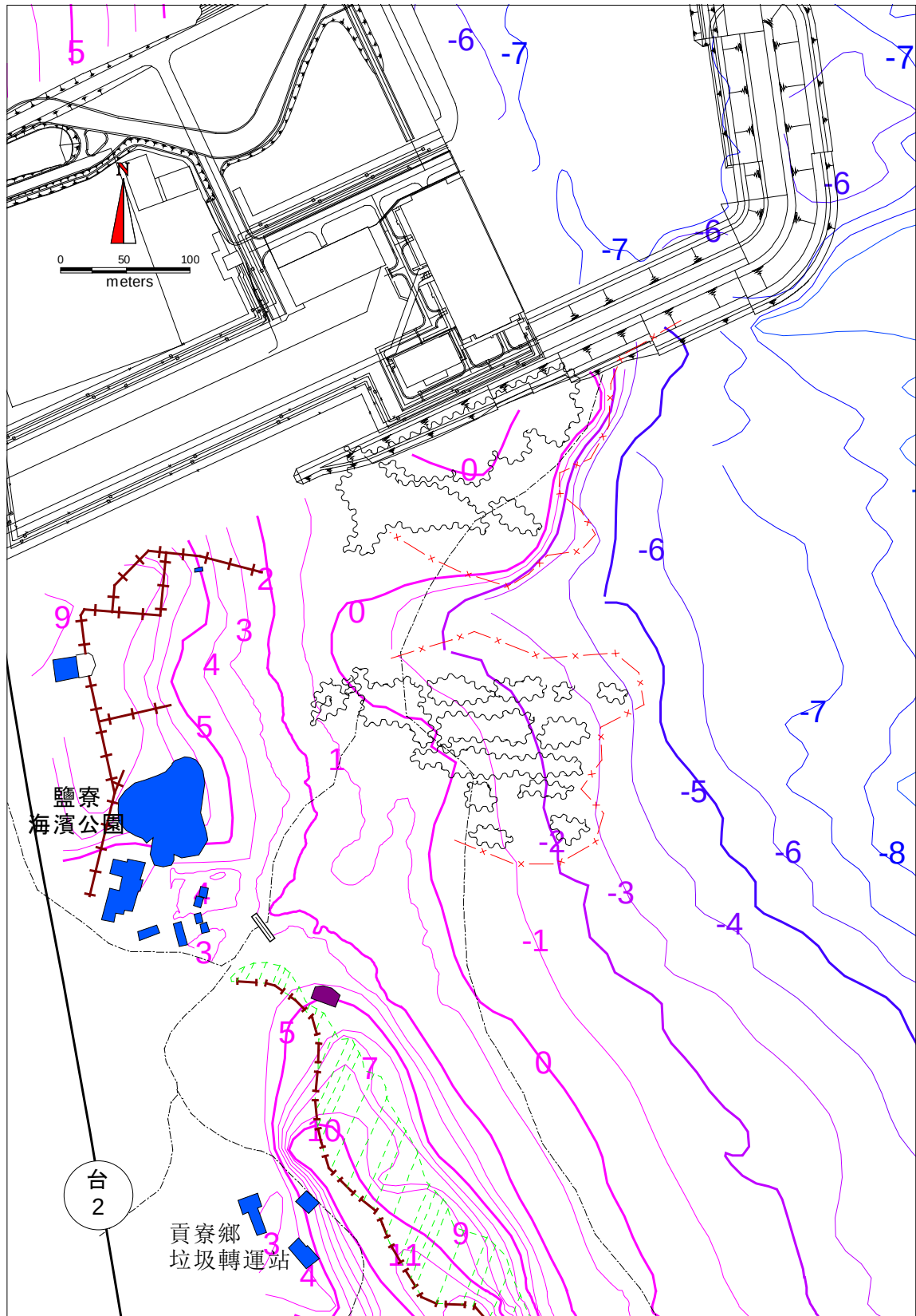
圖 2.5-3 核四封存期間鹽寮公園附近 108 年第 2 季 海岸地形監測結果
