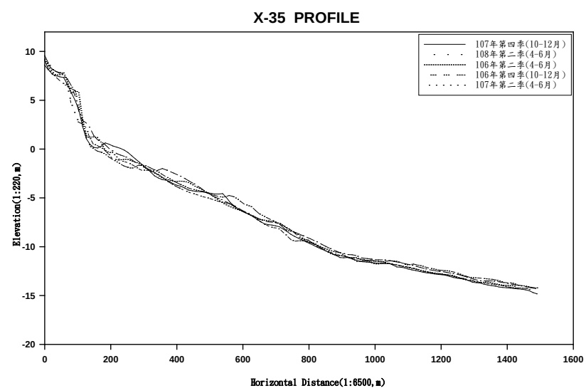
附錄IV.5-3 106年第2季、106年第四季、107年第2季、107年第四季、108年第2季海域監測剖面比較圖(續6)
