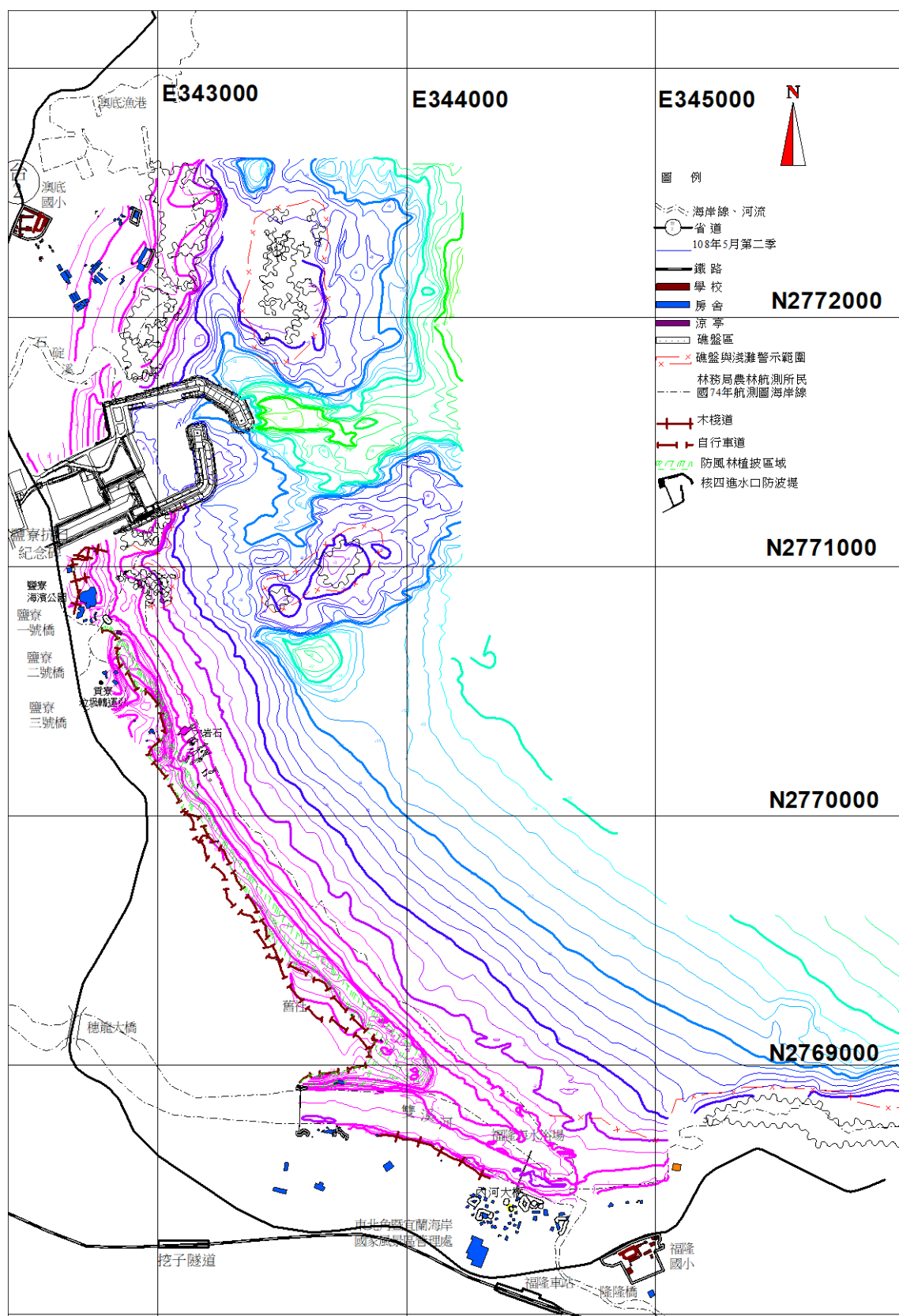
圖 2.5-2 核四封存期間境監測海岸地形 108 年第 2 季 海岸地形監測結果
