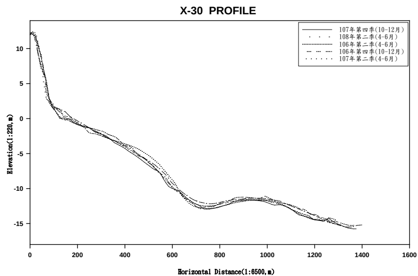
附錄IV.5-3 106年第2季、106年第4季、107年第2季、107年第4季、108年第2季海域監測剖面比較圖(續5)
