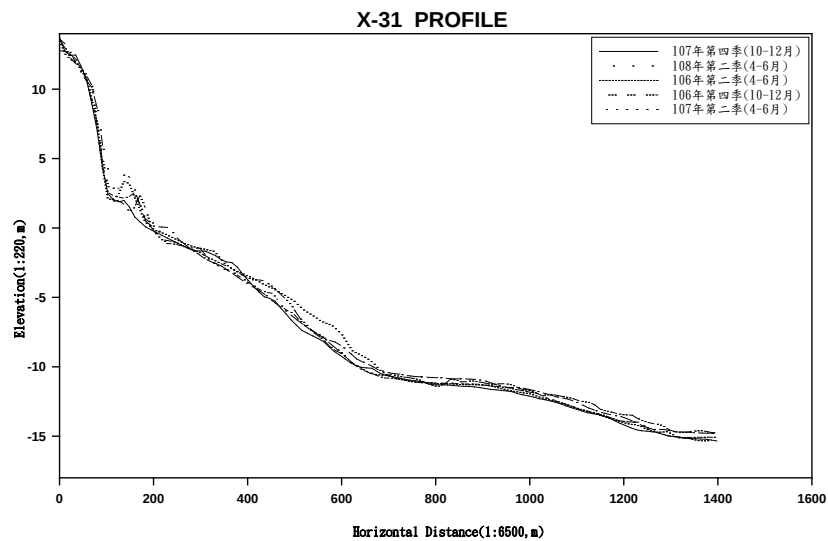
附錄IV.5-3 106年第2季、106年第4季、107年第2季、107年第4季、108年第2季海域監測剖面比較圖(續5)
