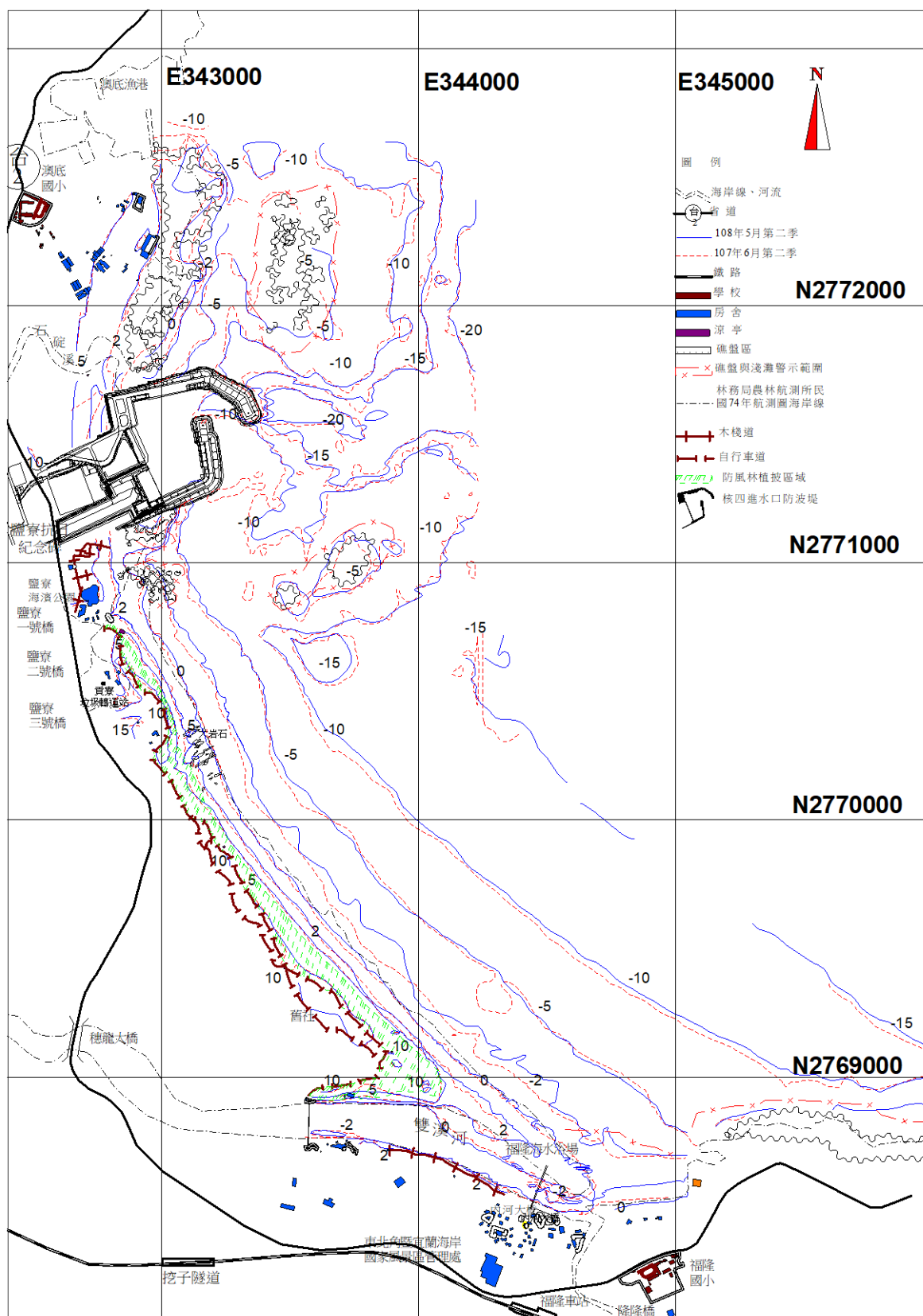
圖 3.1-10 核四環境監測海岸地形 108 年第 2 季與 107 年第 2 季 監測結果比較
