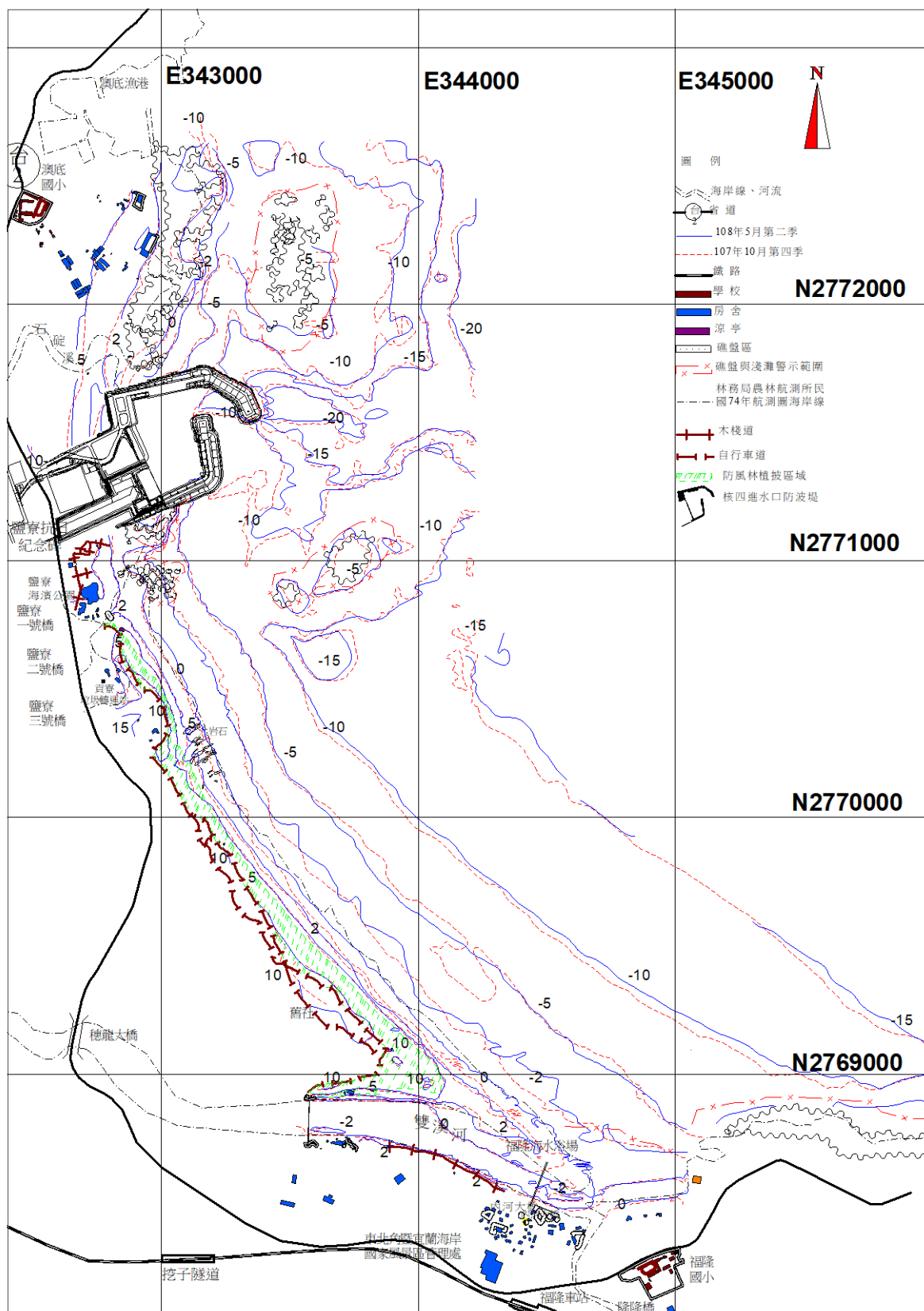
圖 2.5-5 核四封存期間海岸地形 108 年第 2 季與 107 年第 4 季監測結果比較
