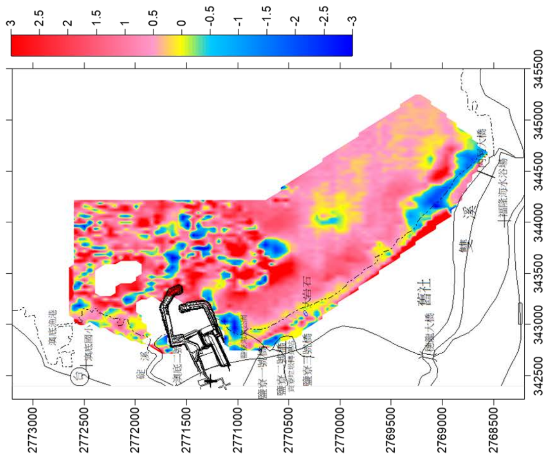
圖 3.1-17核四環境監測海岸地形108年第2季與 87年第2季侵淤比較圖
