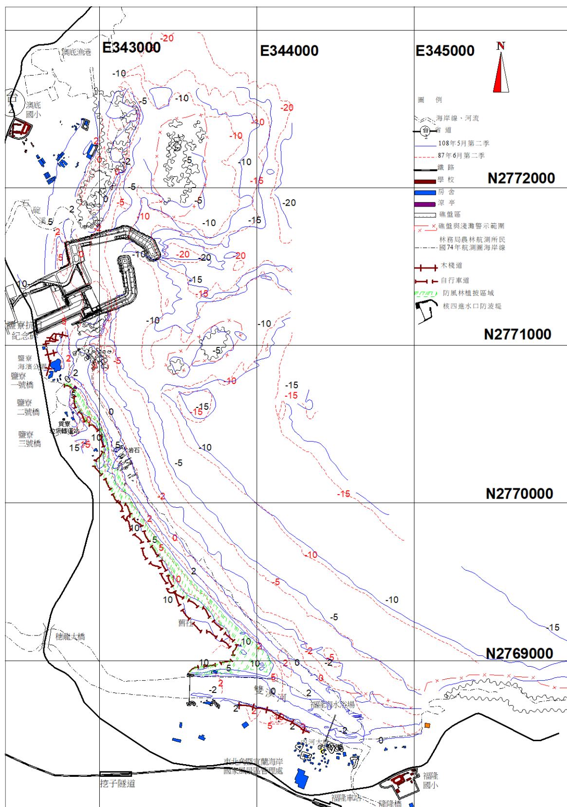
圖 3.1-13 核四環境監測海岸地形 108 年第 2 季與 87 年第 2 季 (海事工程施工前) 監測結果比較
