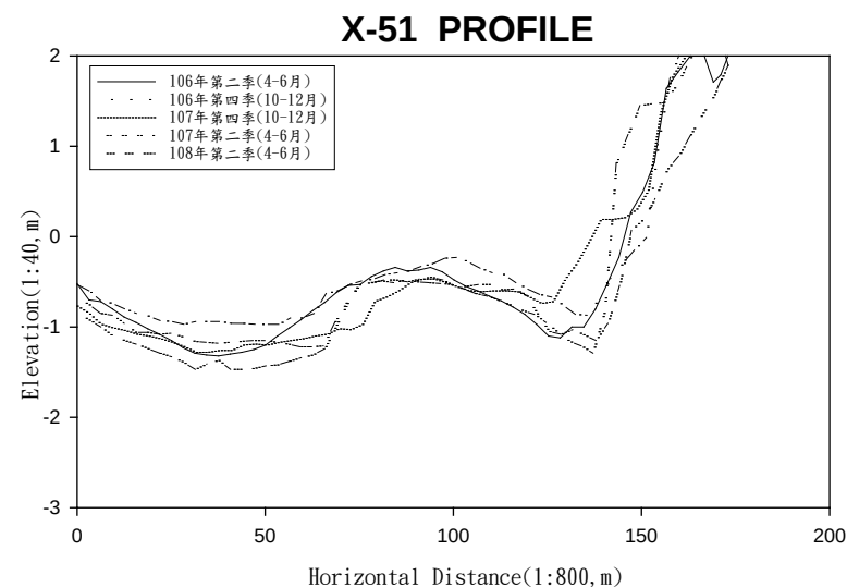
附錄IV.5-3 106年第二季、106年第四季、107年第二季、107年第四季、108年第二季海域監測剖面比較圖(續10)
