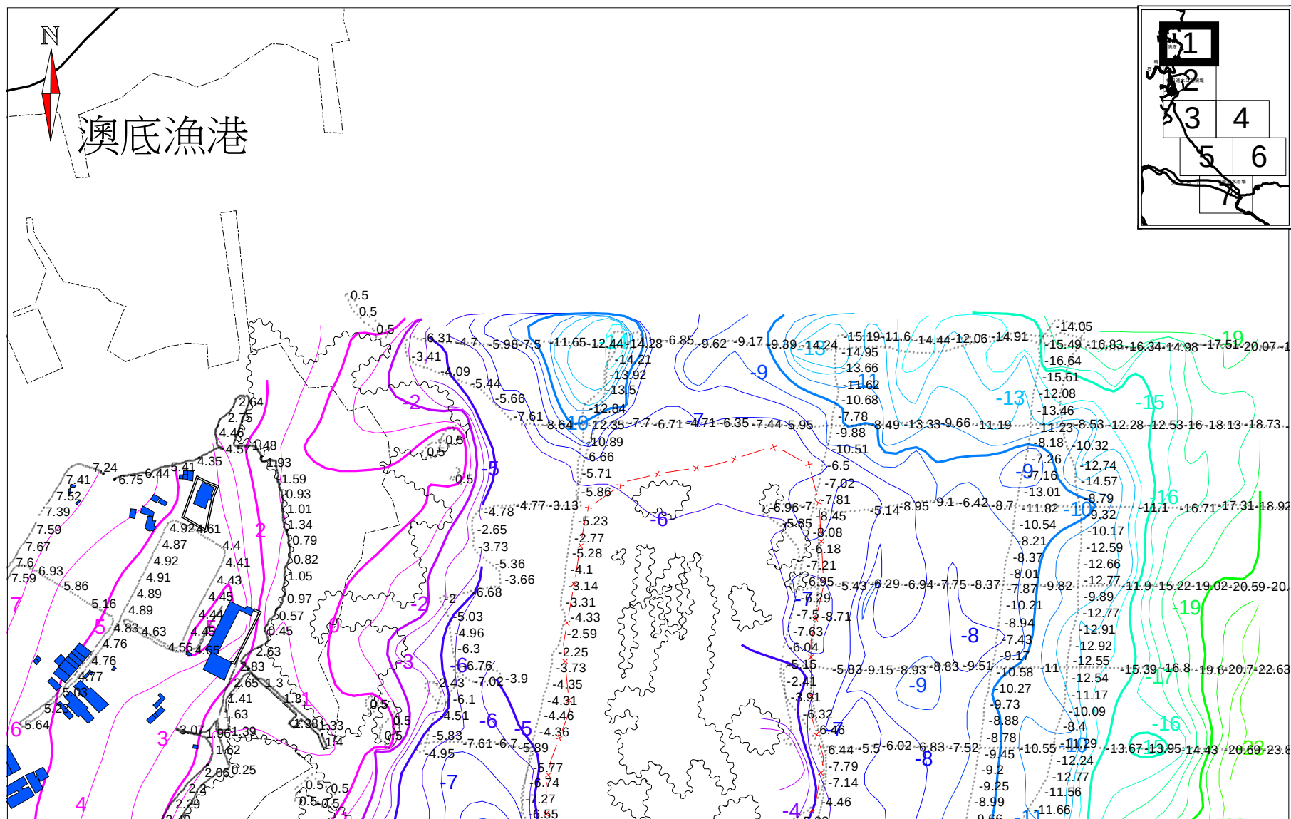
附錄IV.5-2 海岸地形108年5月（第2季）陸域地形、海域地形及水深測量
