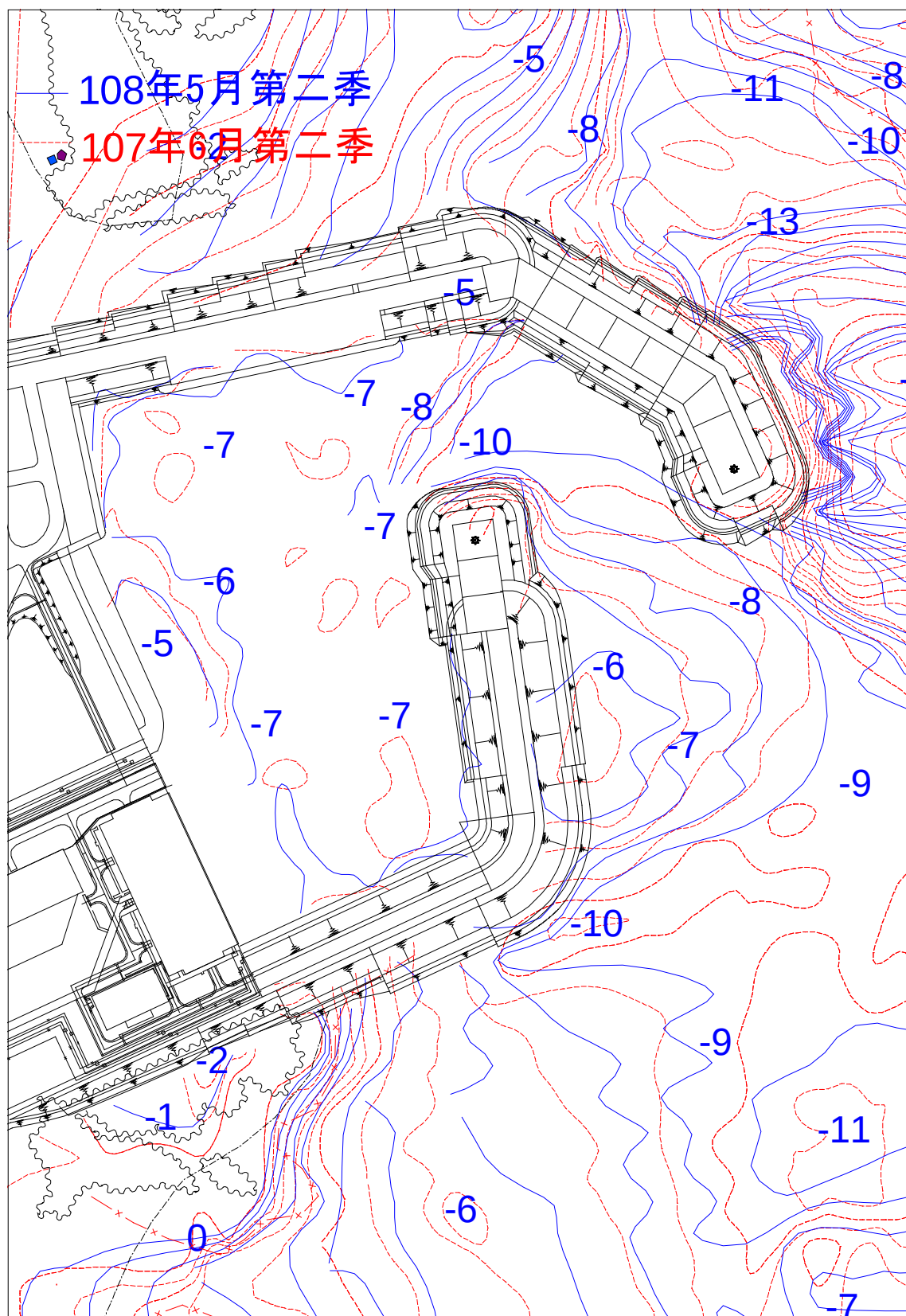
圖 3.1-11 核四環境監測海岸地形進水口防坡堤 108 年第 2 季與 107 年第 2 季監測結果比較
