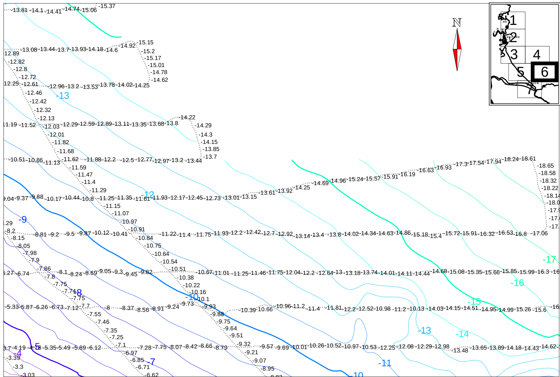
附錄IV.5-2 海岸地形108年5月（第2季）陸域地形、海域地形及水深測量（續5）
