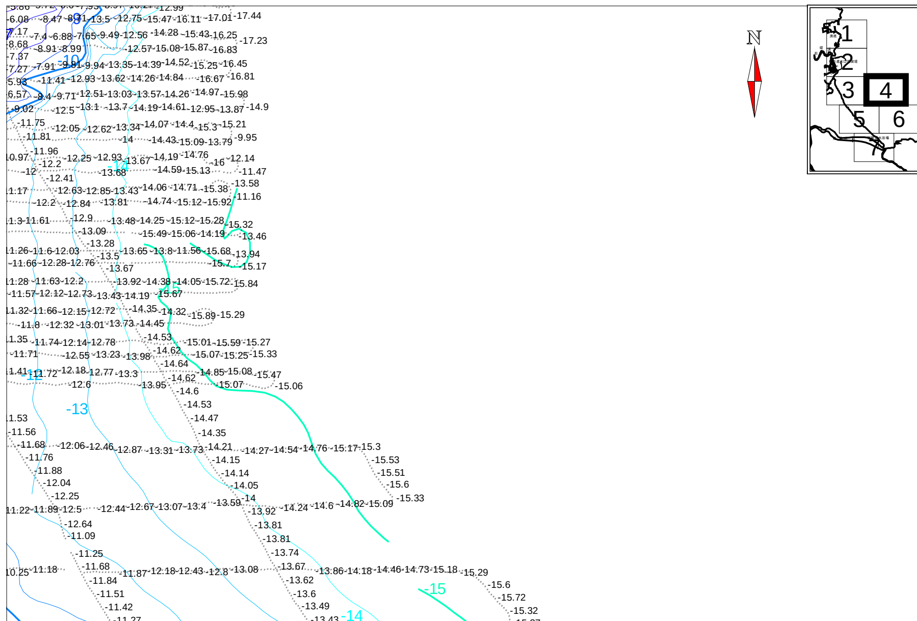
附錄IV.5-2 海岸地形108年5月（第2季）陸域地形、海域地形及水深測量（續3）
