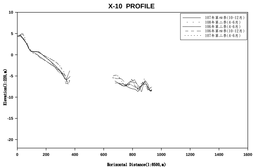
附錄IV.5-3 106年第2季、106年第四季、107年第2季、107年第四季、108年第2季海域監測剖面比較圖
