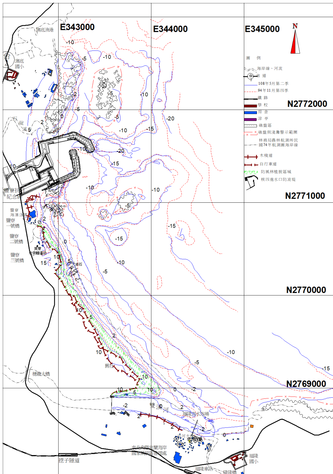
圖 3.1-14 核四環境監測海岸地形 108 年第 2 季與 94 年第 4 季 (海事工程完工後) 監測結果比較
