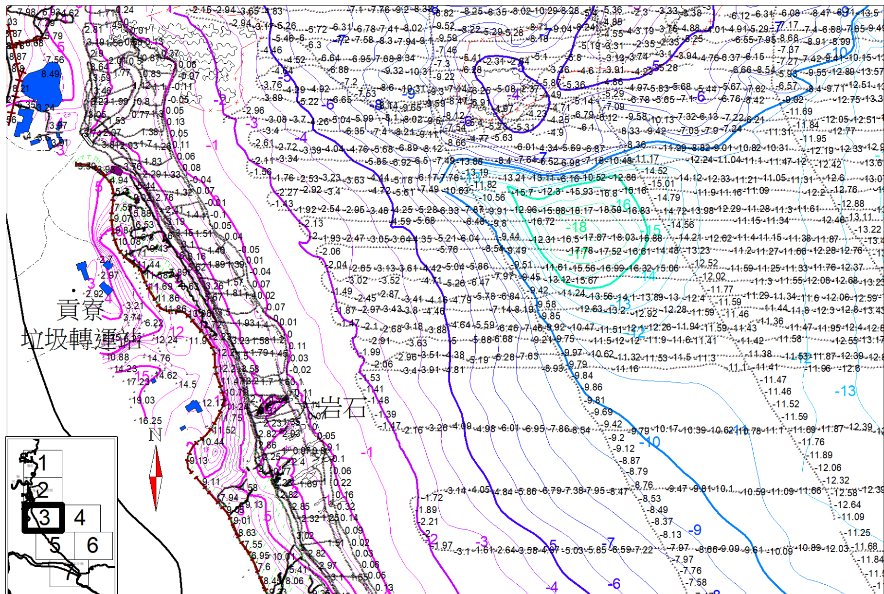
附錄IV.5-2 海岸地形108年5月（第2季）陸域地形、海域地形及水深測量（續2）
