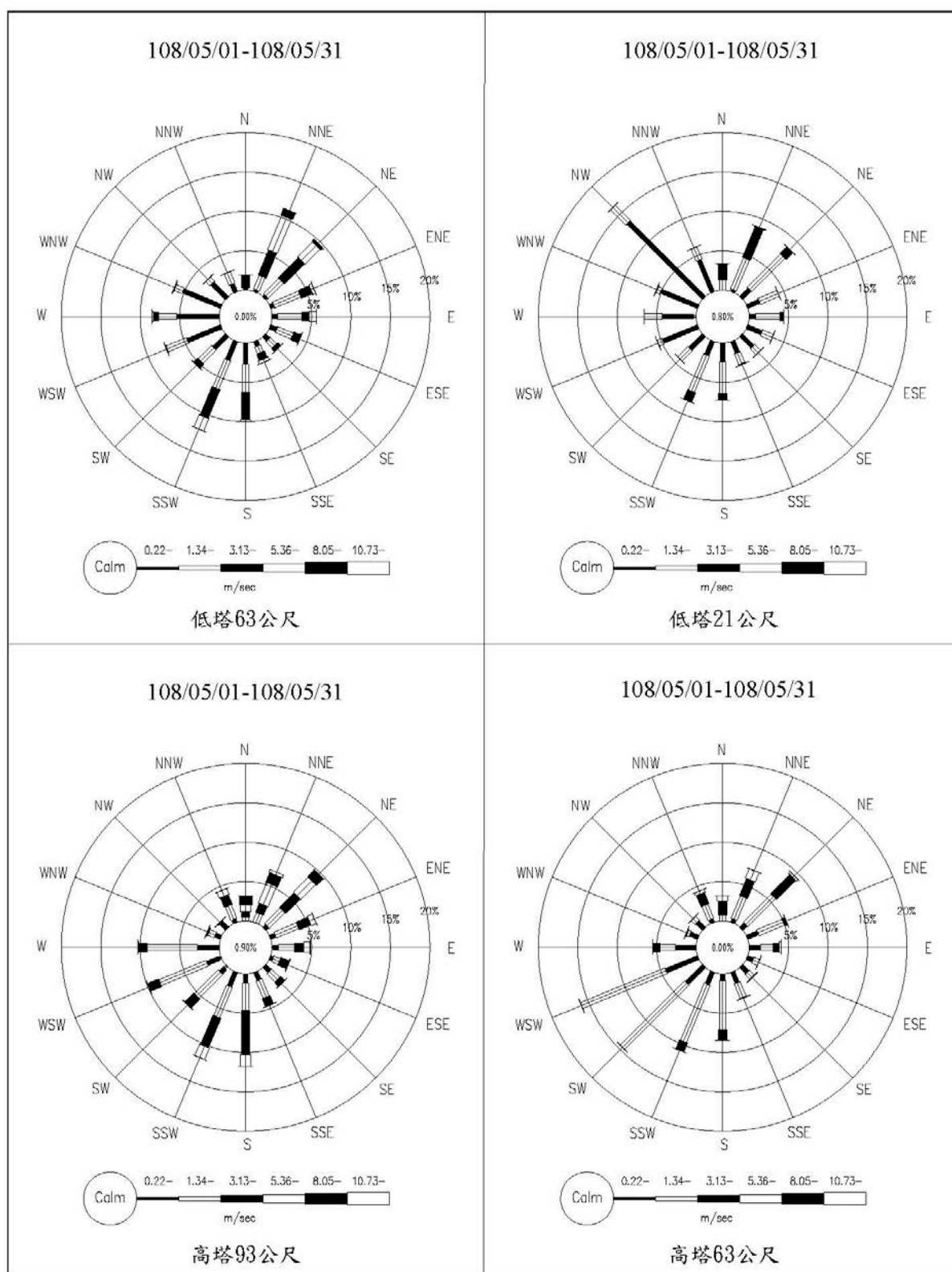
圖 2.1-2 核四封存期間環境監測氣象塔 108 年 5 月風花圖
