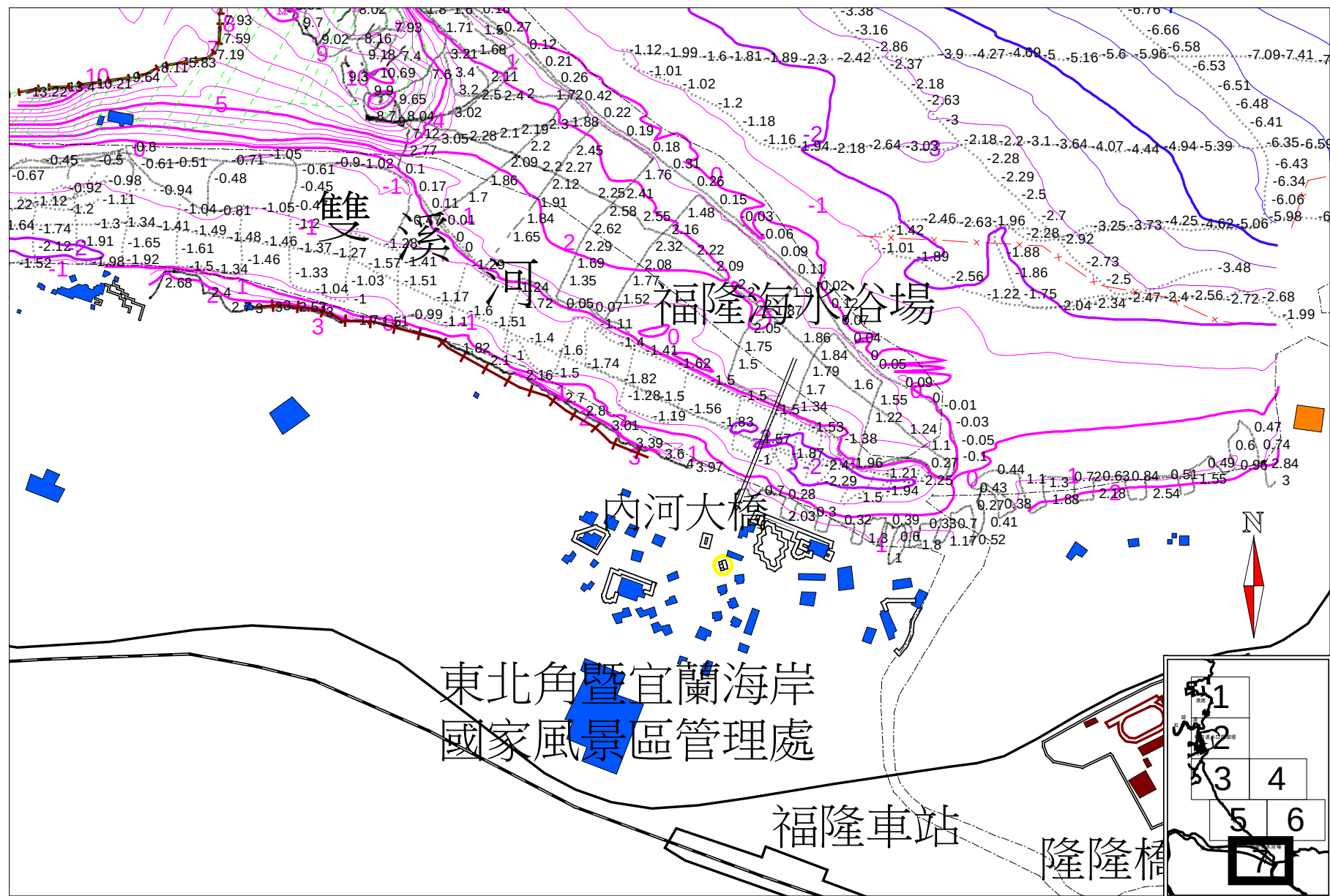
附錄IV.5-2 海岸地形108年5月（第2季）陸域地形、海域地形及水深測量（續6）
